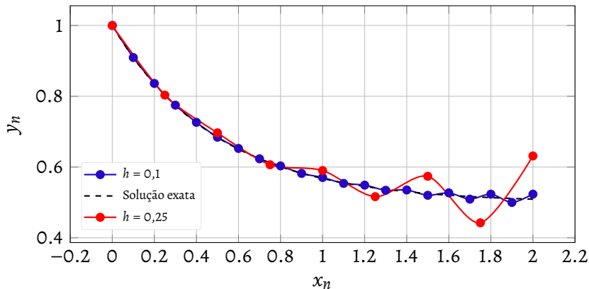
Figura 18 – Comportamento da sequência \{y_n\} para diferentes passos h . Em h = 0,1 a contaminação da raiz espúria ainda não domina no intervalo mostrado; em h = 0,25 ela já é visível. A solução analítica y(x) = \frac{1}{2}(1 + e^{-2x}) está representada pela curva tracejada.
