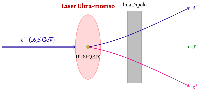
Figura 4 – Esquema do experimento LUXE: colisão entre elétrons de 16,5 GeV e um laser ultra-intenso no ponto de interação (IP). Após a interação, um ímã dipolo separa os produtos — elétrons espalhados ( e^- ), fótons ( \gamma ) e pósitrons ( e^+ ) — permitindo sua detecção independente.
