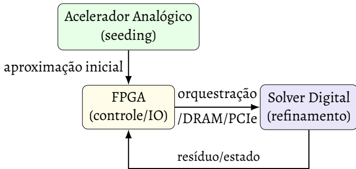
Figura 11 – Papel do FPGA no fluxo híbrido: orquestração entre seeding analógico e refinamento digital.
