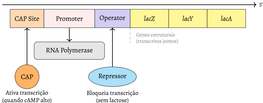
Figura 13 – Representação esquemática do operon lac em E. coli . O sítio CAP ativa a transcrição quando os níveis de cAMP estão elevados (baixa glicose). O repressor LacI liga-se ao operador na ausência de lactose, bloqueando fisicamente a RNA polimerase e impedindo a transcrição dos genes lacZ , lacY e lacA .
