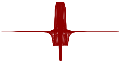
(b) Visão lateral mostrando que o campo elétrico torna-se praticamente nulo a partir de uma certa distância do centro, o que garante a neutralidade elétrica do átomo de hidrogênio.
