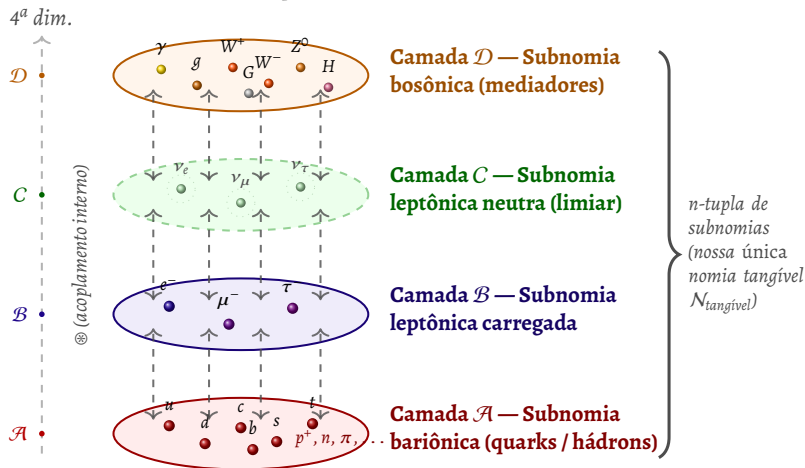
Figura 58 – Representação esquemática da nossa nomia tangível \mathcal{N}_{\text{tangível}} como uma n-tupla de subnomias , dispostas em camadas ontológicas distintas: \mathcal{A} (bariônica), \mathcal{B} (leptônica carregada), \mathcal{C} (leptônica neutra, no limiar) e \mathcal{D} (bosônica). As setas tracejadas verticais representam o acoplamento \otimes entre subnomias, codificando a estrutura \mathcal{K} = (\mathcal{M}, \mathcal{R}, \mathcal{A}) de mistura, representação compartilhada e condições de anomalia (Capítulo 14). Observação crucial: os discos NÃO representam realidades paralelas independentes, mas sim setores (subnomias) da mesma nomia tangível , acoplados internamente. A interação próton–elétron (Figuras 54 e 55) manifesta-se como o acoplamento \mathcal{A} \otimes \mathcal{B} .
