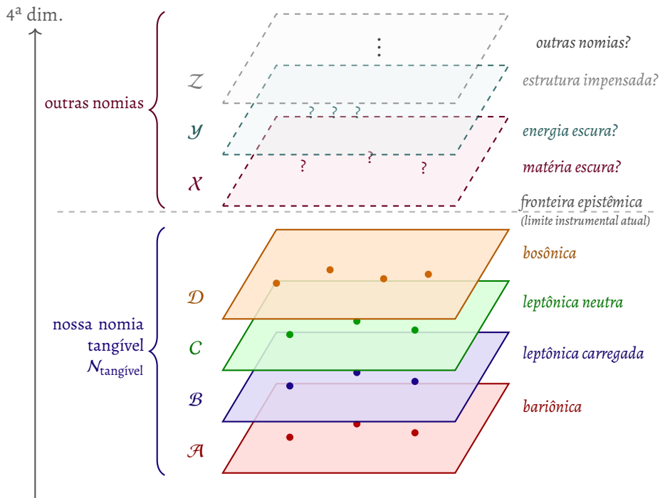
Figura 59 – Extensão especulativa da representação em camadas ao longo da quarta dimensão (cf. Figura 57). Abaixo da fronteira epistêmica, empilham-se as quatro subnomias da nossa nomia tangível \mathcal{N}_{\text{tangível}} : \mathcal{A} (bárionica), \mathcal{B} (leptônica carregada), \mathcal{C} (leptônica neutra) e \mathcal{D} (bosônica) — camadas sólidas , detectáveis pelos instrumentos atuais. Acima da fronteira epistêmica (linha tracejada horizontal), camadas tracejadas e progressivamente esmaecidas representam nomias hipotéticas: \mathcal{X} poderia corresponder, especulativamente, à matéria escura; \mathcal{Y} , à energia escura; \mathcal{Z} e as camadas acima representam estruturas ainda impensadas ou inacessíveis. A fronteira epistêmica é histórica e instrumental : caso partículas fundamentais hoje desconhecidas venham a ser descobertas, adotamos, por convenção, que elas habitarão camadas distintas de \mathcal{A} , \mathcal{B} , \mathcal{C} , \mathcal{D} — ou seja, fora da nomia tangível tal como definida neste livro. Esta figura não representa realidades paralelas no sentido de Everett: as camadas aqui ilustradas coexistem na mesma 4ª dimensão, mas são mutuamente inacessíveis aos instrumentos típicos de cada nomia.
