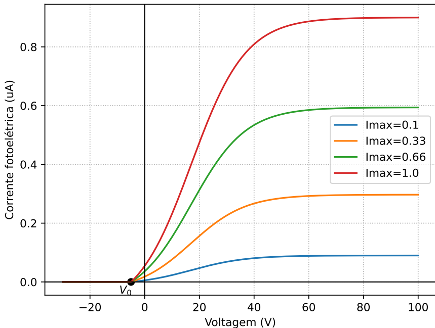
Figura 13 – Corrente fotoelétrica em função da voltagem para diferentes intensidades de luz com mesma frequência.
