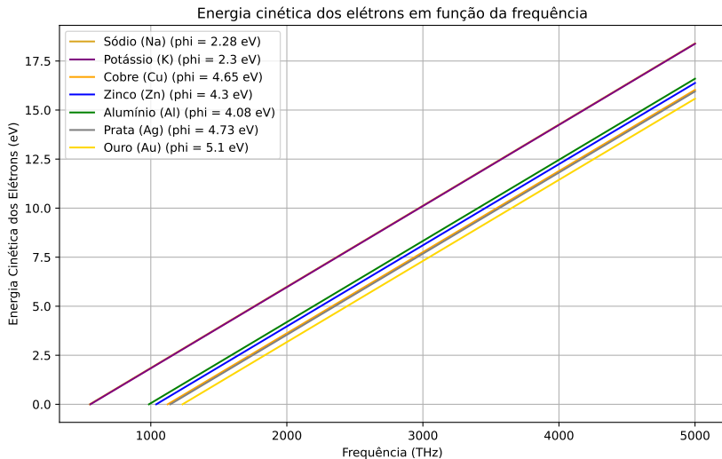
Figura 14 – Energia cinética dos fotoelétrons emitidos em função da frequência da luz para diferentes metais.
