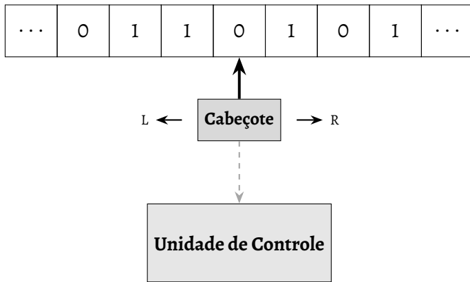
Figura 15 – Representação esquemática de uma Máquina de Turing. O modelo consiste em uma fita potencialmente ilimitada dividida em células, cada uma contendo um símbolo. O cabeçote lê e escreve símbolos na fita, podendo mover-se para a esquerda (L) ou direita (R). A unidade de controle determina a ação a ser executada com base no estado atual e no símbolo lido, definindo o próximo estado, o símbolo a ser escrito e a direção do movimento.
