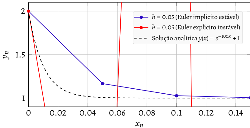
Figura 19 – Rigidez numérica na equação y' = -100y + 100 , y(0) = 2 , com mesmo passo h = 0,05 em dois métodos distintos. O método de Euler explícito (curva vermelha) é numericamente instável e gera valores que explodem em magnitude e trocam de sinal a cada iteração. Já o método de Euler implícito (curva azul) permanece estável e aproxima-se rapidamente de y = 1 , em acordo com a solução analítica (curva tracejada). Este contraste mostra por que problemas rígidos exigem métodos implicitamente estáveis.
