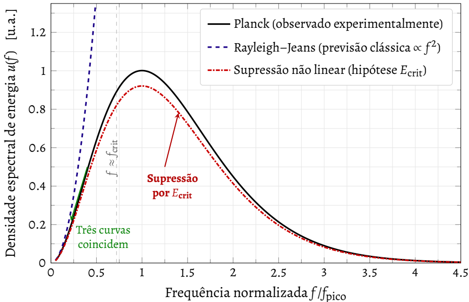
Figura 8 – Comparação qualitativa entre a previsão clássica de Rayleigh-Jeans (tracejada azul, u \propto f^2 , divergente), a distribuição de Planck observada experimentalmente (sólida preta) e o comportamento pretendido pela hipótese de supressão não linear (traço-ponto vermelha; ilustração, não resultado de cálculo a partir da hipótese). Quando o campo elétrico dos modos de alta frequência atinge E_{\text{crit}} , a não linearidade restitutiva impede o acúmulo indefinido de energia, produzindo um corte natural nas altas frequências qualitativamente compatível com a curva de Planck. Compare com a Figura 12 do Apêndice Q.
