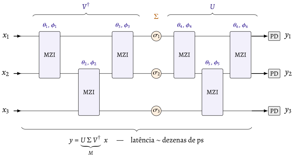
Figura 12 – Esquema conceitual de um solucionador fotônico one-shot 3 \times 3 baseado na decomposição SVD. As três linhas horizontais representam guias de onda. Cada retângulo “MZI” é um interferômetro de Mach–Zehnder que acopla dois guias adjacentes por meio de defasadores (\theta, \phi) ; os círculos \sigma_i são atenuadores ópticos que implementam os valores singulares; e “PD” denota fotodetectores de saída.
