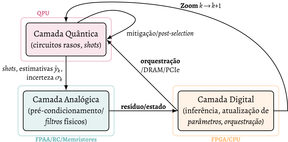
Figura 9 – Arquitetura tri-híbrida da metacamada quântico-clássica do MZS.
