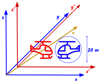
Figura 22 – Dois helicópteros tridimensionais 1 sobrevoando os seus respectivos espaços 3D, mas cada espaço (ou universo) está afastado um do outro por alguns nanômetros ao longo da quarta dimensão v . O tamanho dos helicópteros é tal que eles caberiam numa esfera de 20 metros de diâmetro.
