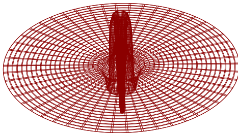
(a) Modelo simplista de um átomo de hidrogênio.
