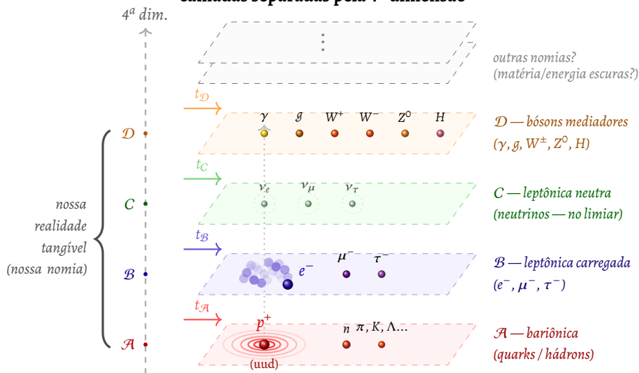
Figura 58 – Representação ontológica em camadas das subnomias que compõem a nossa nomia (realidade tangível). Cada camada corresponde a uma subnomia distinta, separada das demais pela quarta dimensão. Na camada bariônica \mathcal{A} , o próton p^+ (composto de quarks uud ) gera um campo elétrico com perfil radial característico. Na camada leptônica carregada \mathcal{B} , o elétron e^- ocupa uma posição específica — desconhecida para um observador da camada \mathcal{A} —, representada pela nuvem de ignorância (sombas azuis) concentrada em torno da projeção vertical do próton, dando origem ao orbital 1s . A camada \mathcal{C} (neutrinos) situa-se no limiar da nossa nomia, quase desacoplada das demais subnomias. A camada \mathcal{D} abriga os bósons mediadores das interações fundamentais. Cada camada possui sua própria estrutura temporal ( t_A, \dots, t_D ), desconectada das demais. Acima da chave estão indicadas, de forma hipotética, outras nomias eventualmente não detectáveis por nossos instrumentos — possivelmente associadas à matéria e à energia escuras.
