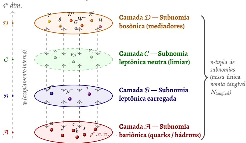
Figura 59 – Representação esquemática da nossa nomia tangível \mathcal{N}_{\text{tangível}} como uma n-tupla de subnomias , dispostas em camadas ontológicas distintas: \mathcal{A} (bariônica), \mathcal{B} (leptônica carregada), \mathcal{C} (leptônica neutra, no limiar) e \mathcal{D} (bosônica). As setas tracejadas verticais representam o acoplamento \otimes entre subnomias, codificando a estrutura \mathcal{C} = (\mathcal{M}, \mathcal{R}, \mathcal{A}) de mistura, representação compartilhada e condições de anomalia (Capítulo 14). Observação crucial: os discos NÃO representam realidades paralelas independentes, mas sim setores (subnomias) da mesma nomia tangível , acoplados internamente. A interação próton–elétron (Figuras 54 e 56) manifestase como o acoplamento \mathcal{A} \otimes \mathcal{B} .
