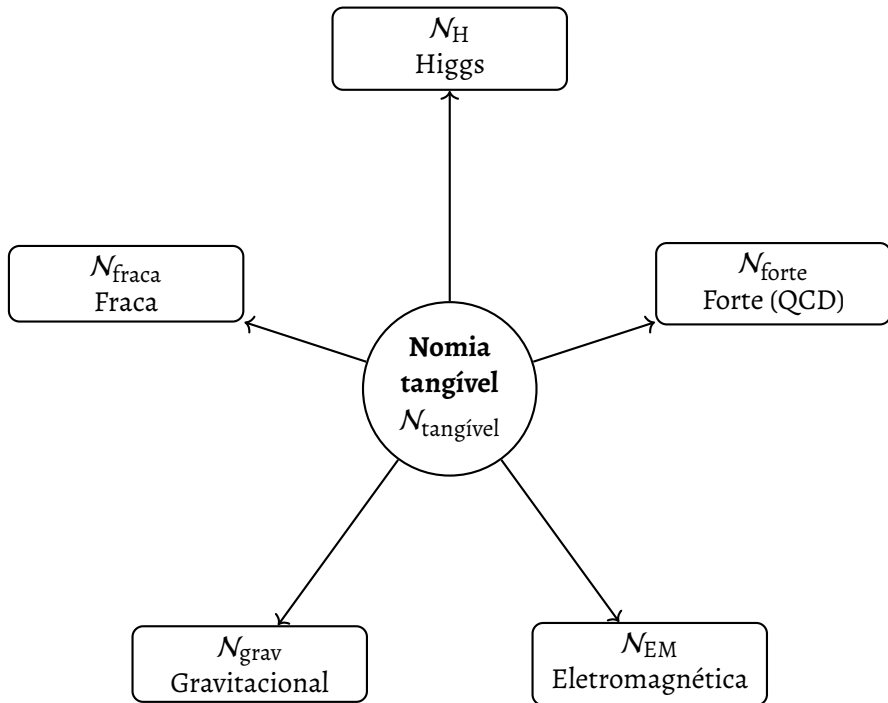
Figura 62 – Estrutura da nomia da nossa realidade tangível como composição das cinco subnomias fundamentais: de Higgs, fraca, forte, gravitacional e eletromagnética.
