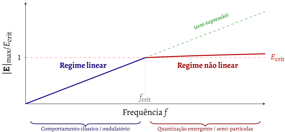
Figura 11 – Diagrama esquemático da amplitude máxima do campo elétrico em função da frequência, para uma dada amplitude de potencial V_0 . No regime linear ( f < f_{\text{crit}} ), |\vec{E}| cresce proporcionalmente a f (reta azul). Ao atingir E_{\text{crit}} , a não linearidade restitutiva entra em ação e limita o crescimento do campo (curva vermelha), formando excitações localizadas. A reta tracejada cinza indica o que ocorreria sem supressão.
