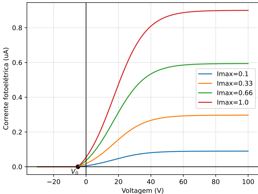
Figura 14 – Corrente fotoelétrica em função da voltagem para diferentes intensidades de luz com mesma frequência.
