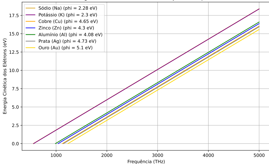
Figura 15 – Energia cinética dos fotoelétrons emitidos em função da frequência da luz para diferentes metais.
