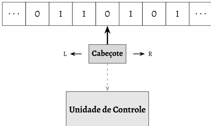
Figura 16 – Representação esquemática de uma Máquina de Turing. O modelo consiste em uma fita infinita dividida em células, cada uma contendo um símbolo. O cabeçote lê e escreve símbolos na fita, podendo mover-se para a esquerda (L) ou direita (R). A unidade de controle determina a ação a ser executada com base no estado atual e no símbolo lido, definindo o próximo estado, o símbolo a ser escrito e a direção do movimento.
