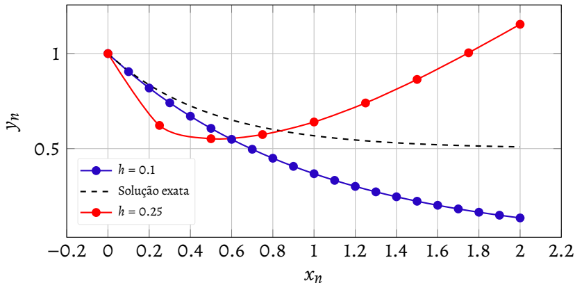
Figura 18 – Comportamento da sequência \{y_n\} para diferentes passos h . O método é estável para h = 0.1 e torna-se instável para h = 0.25 . A solução analítica y(x) = \frac{1}{2}(1 + e^{-2x}) está representada pela curva tracejada.
