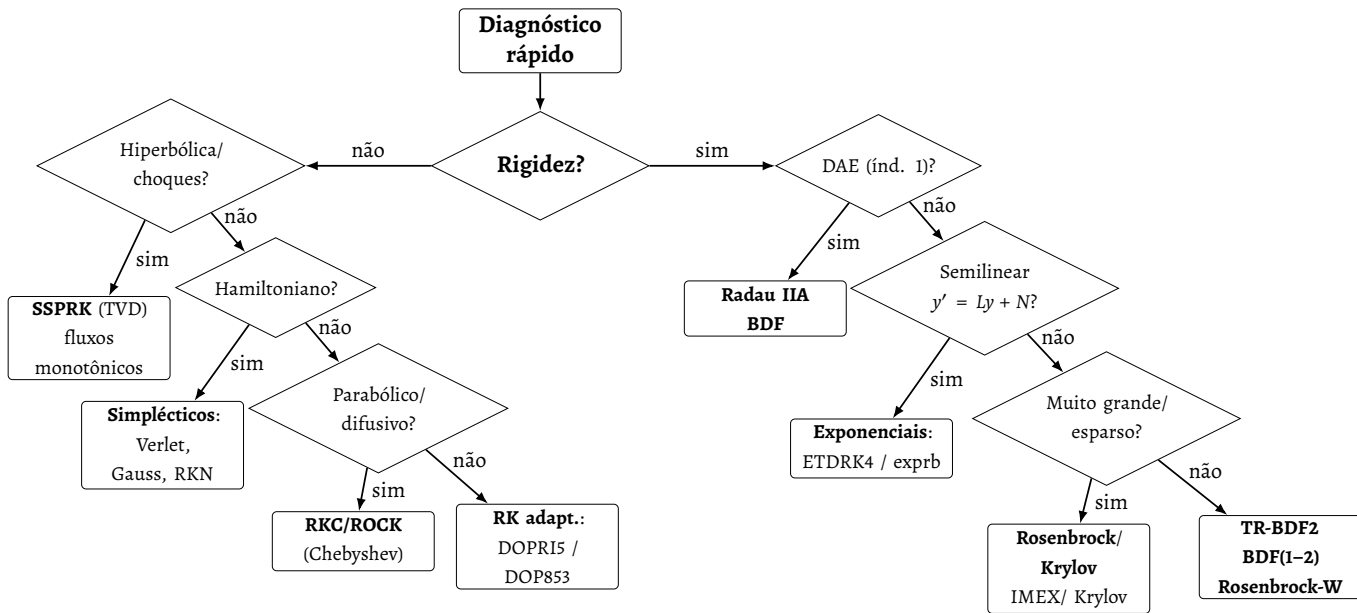
Figura 21 – Mapa de escolha (fluxograma) do algoritmo numérico mais indicado a ser utilizado para resolver o problema de resolução de ODEs, partindo-se da identificação da rigidez do problema.
