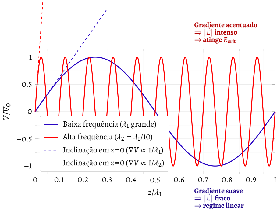
Figura 7 – Comparação do potencial elétrico V(z) para duas ondas com a mesma amplitude V_0 , porém com frequências diferentes, no instante t = 0 . A onda de alta frequência (vermelha, \lambda_2 = \lambda_1/10 ) apresenta um gradiente espacial 10 vezes mais acentuado que a onda de baixa frequência (azul). Pela relação \vec{E} = -\nabla V , isso resulta em um campo elétrico 10 vezes mais intenso. É precisamente este efeito que faz com que os modos de alta frequência atinjam E_{\text{crit}} primeiro, ativando a supressão não linear.
