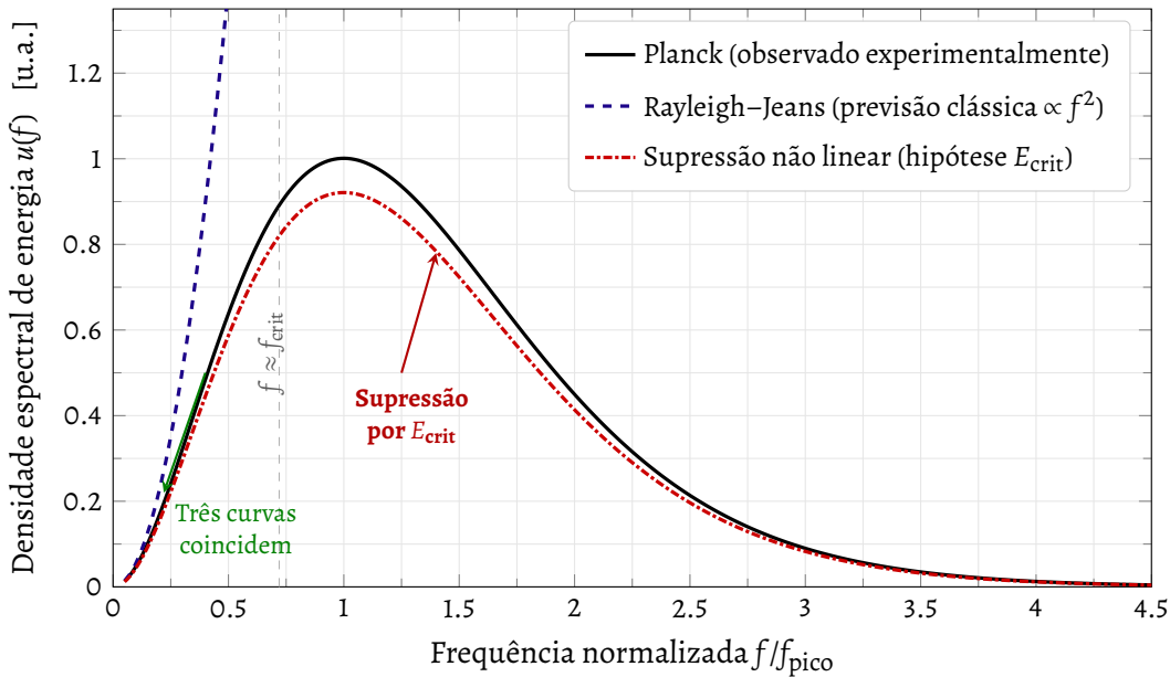
Figura 8 – Comparação qualitativa entre a previsão clássica de Rayleigh-Jeans (tracejada azul, u \propto f^2 , divergente), a distribuição de Planck observada experimentalmente (sólida preta) e o comportamento esperado pela hipótese de supressão não linear (traço-ponto vermelha). Quando o campo elétrico dos modos de alta frequência atinge E_{\text{crit}} , a não linearidade restitutiva impede o acúmulo indefinido de energia, produzindo um corte natural nas altas frequências qualitativamente compatível com a curva de Planck. Compare com a Figura 13 do Apêndice Q.
