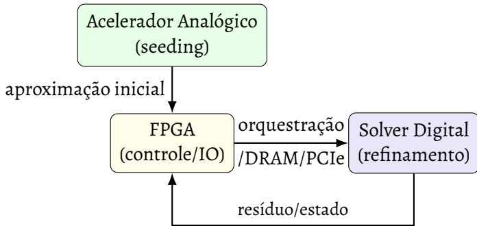
Figura 10 – Papel do FPGA no fluxo híbrido: orquestração entre seeding analógico e refinamento digital.
