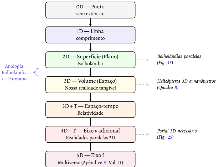
Figura 26 – Hierarquia dimensional: do ponto adimensional ao multiverso 5D. Cada nível adiciona uma coordenada que amplia o espaço de possibilidades. As realidades paralelas da Bolholândia (2D) são análogas às realidades paralelas do nosso espaço (3D), separadas ao longo de um eixo adicional por distâncias que podem ser sub-nanométricas.
