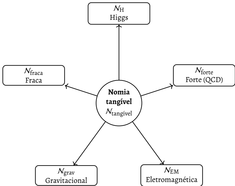
Figura 62 – Estrutura da nomia da nossa realidade tangível como composição das cinco subnomias fundamentais: de Higgs, fraca, forte, gravital e eletromagnética.
