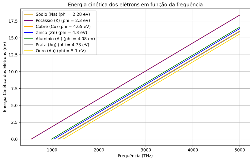
Figura 15 – Energia cinética dos fotoelétrons emitidos em função da frequência da luz para diferentes metais.
