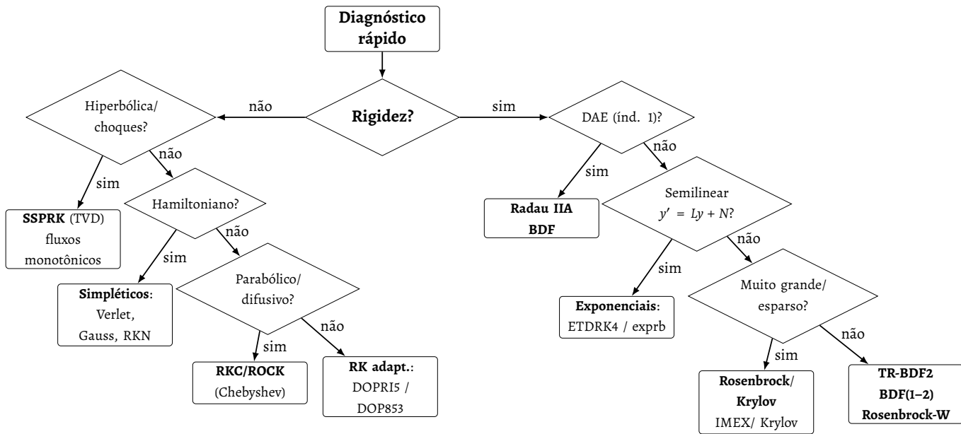
Figura 21 – Fluxograma de escolha do método numérico mais indicado para a integração de ODEs, partindo da identificação da rigidez do problema.
