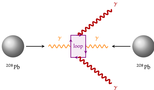
Figura 5 – Espalhamento luz-por-luz ( \gamma\gamma \rightarrow \gamma\gamma ) em colisões ultra-periféricas Pb–Pb no LHC. Cada núcleo relativístico emite um fóton quasi-real; estes interagem via um loop de férmions virtuais (diagrama de box ), produzindo dois fótons reais no estado final (ATLAS Collaboration, 2017; ATLAS Collaboration, 2019).
