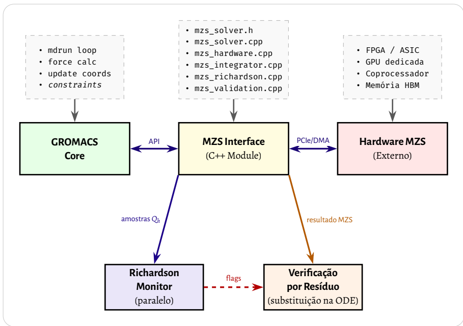
Figura 17 – Arquitetura de integração MZS-GROMACS, incluindo módulos de monitoramento por Richardson e validação numérica.
