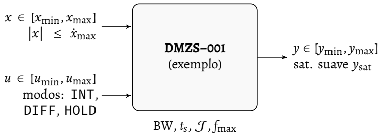
Figura 6 – Diagrama de blocos do DMZS, com entradas, saídas e parâmetros principais.
