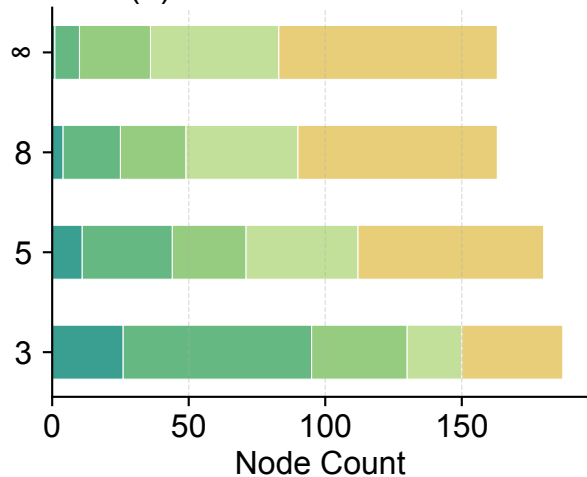
(d) SciWorld — Env Tree
