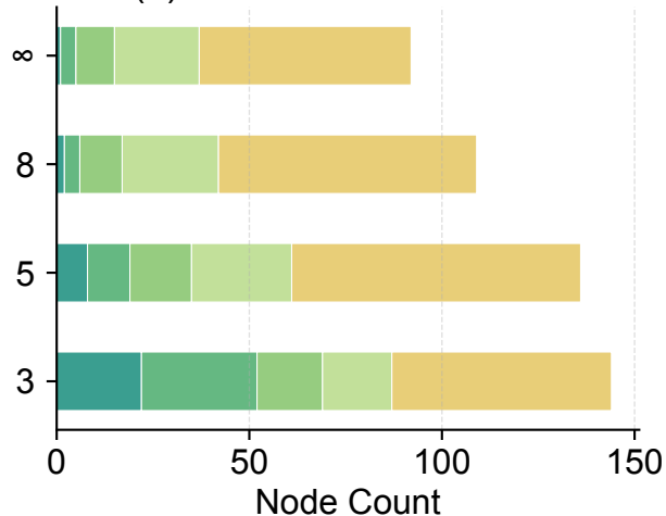
(d) SciWorld — Env Tree
