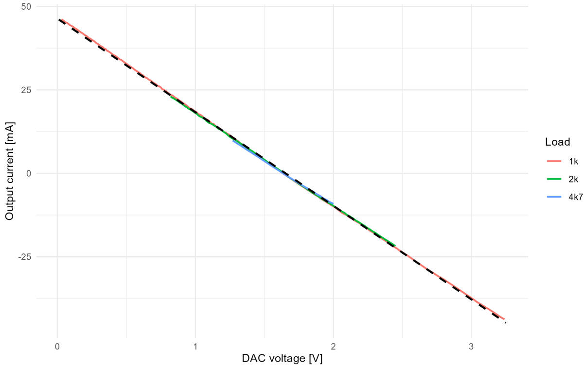
Figura 8: Curvas experimentais de corrente e modelo linear global
