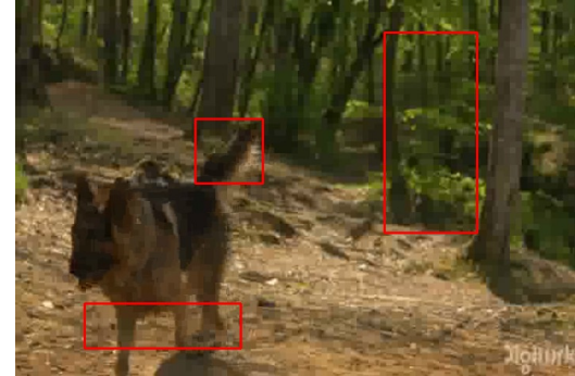
DCVC-HEM (0.0364 / 0.171 / 67.44)
