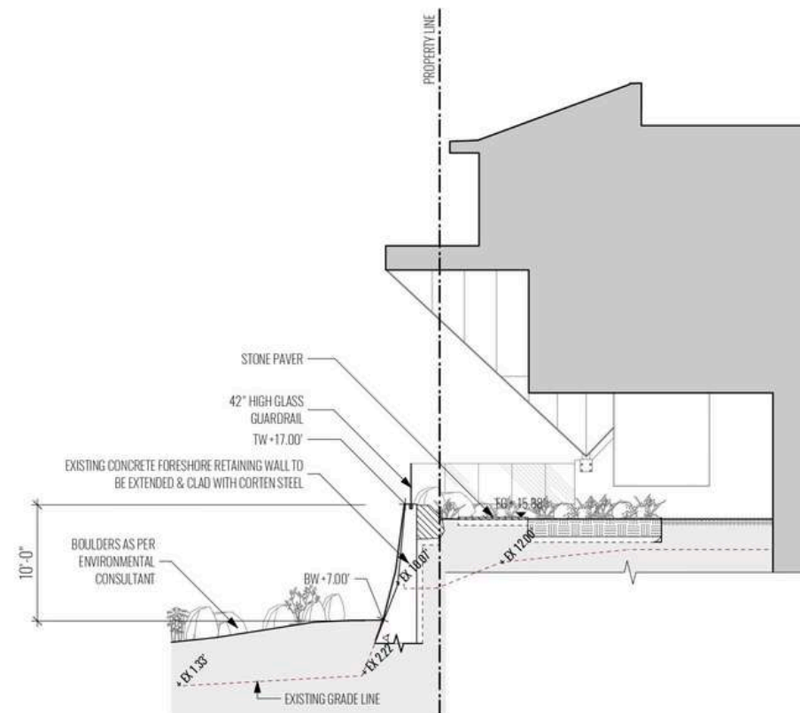
SECTION C Scale: 1/8" = 1' -0"
