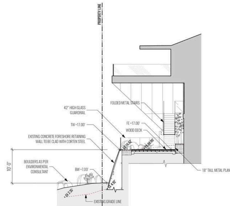
SECTION D Scale: 1/8" = 1' -0"
