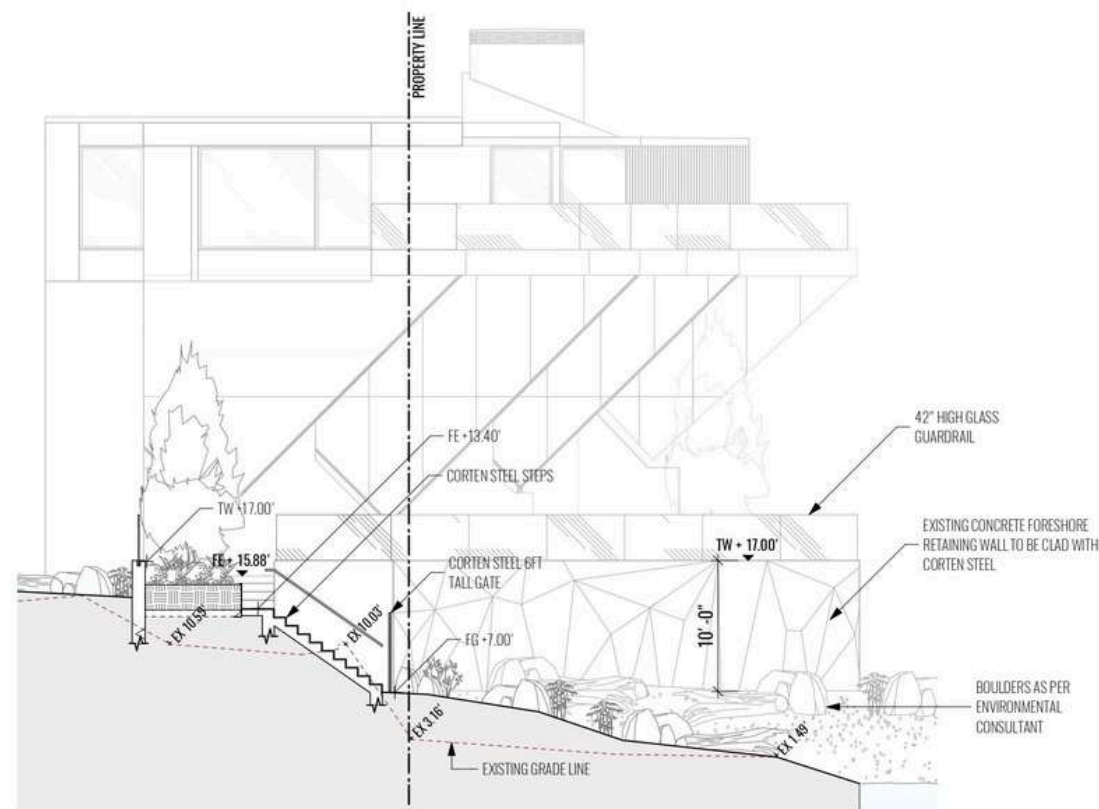
SECTION B Scale: 1/8" = 1' -0"
