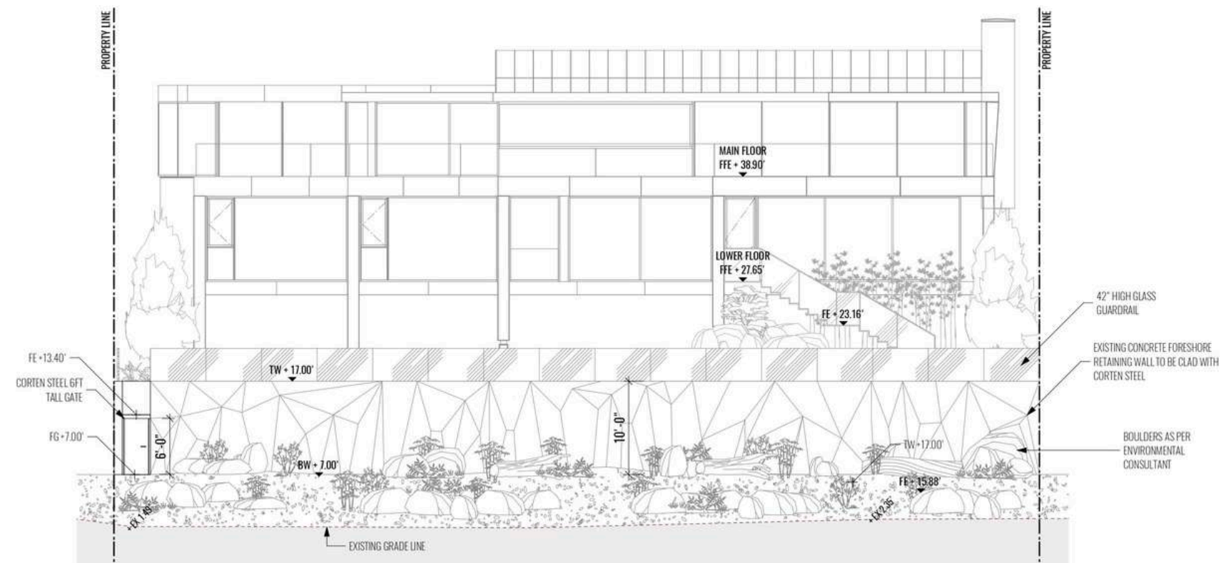
SECTION A Scale: 1/8" = 1' -0"
