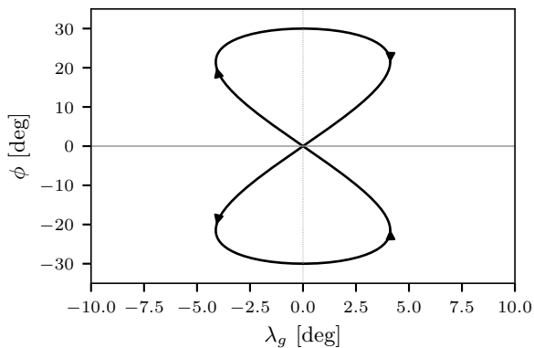
(d) i = 10^\circ , e = 0.4 : distorted (drop) shape
