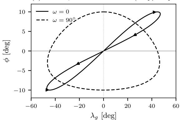
(d) i = 10^\circ , e = 0.4 : distorted (drop) shape
