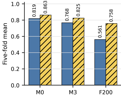
(a) AUPRC
