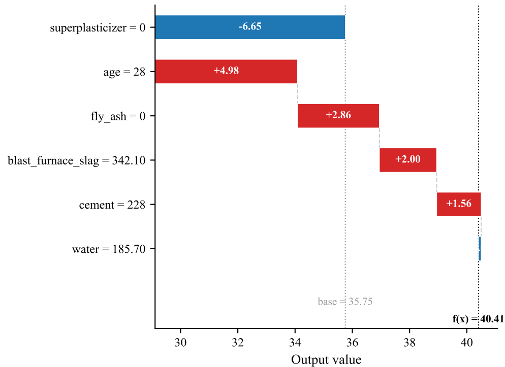
SHAP Values
