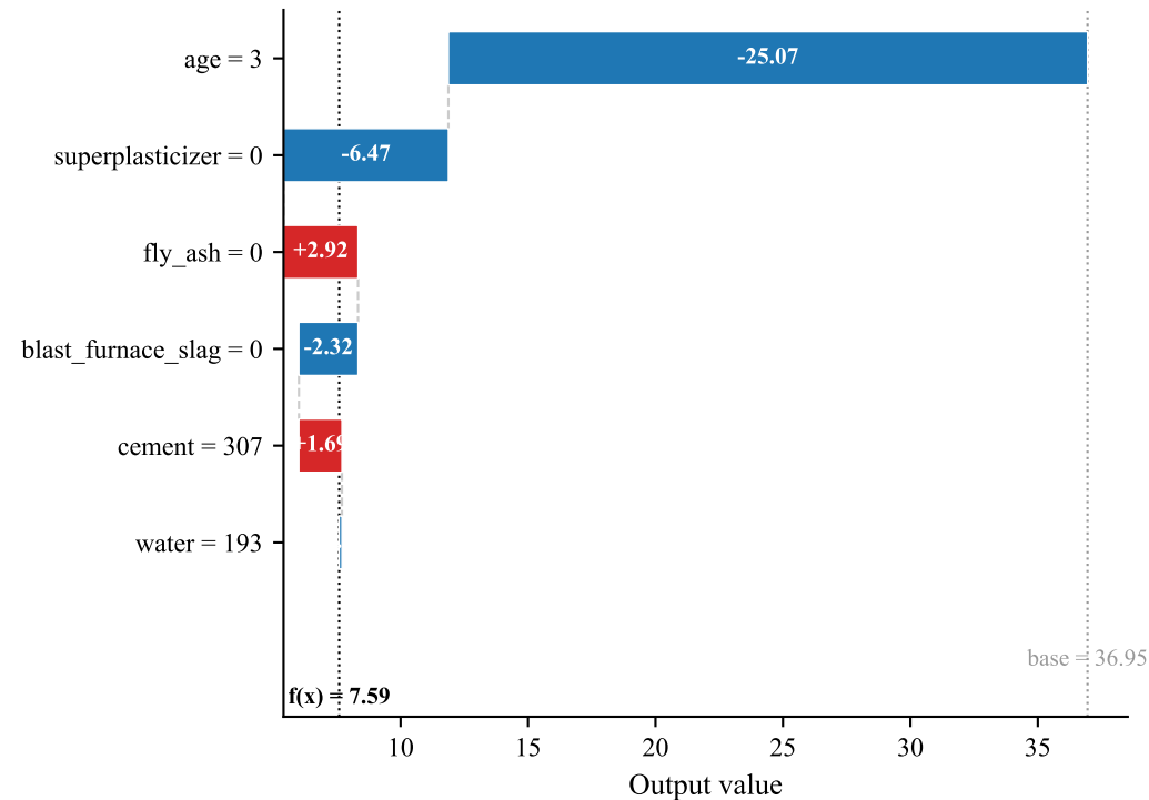
SHAP Values
