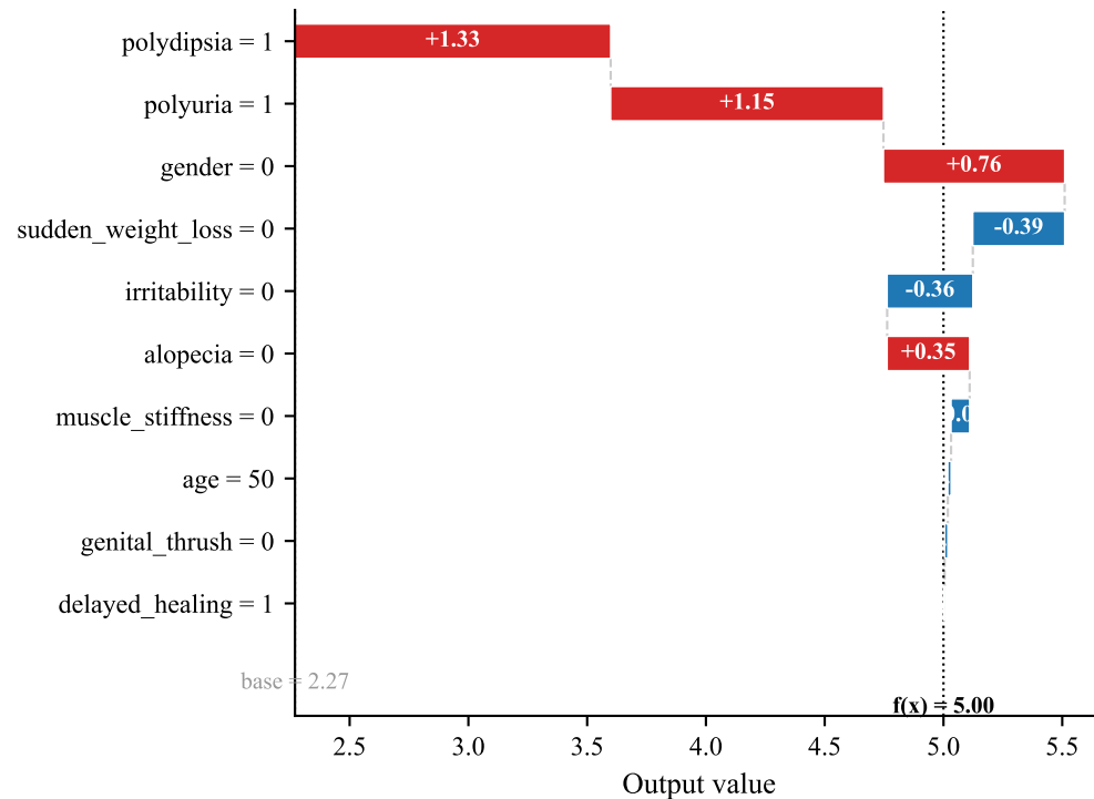
SHAP Values
