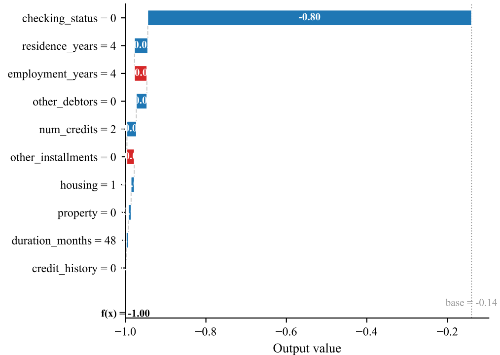
SHAP Values
