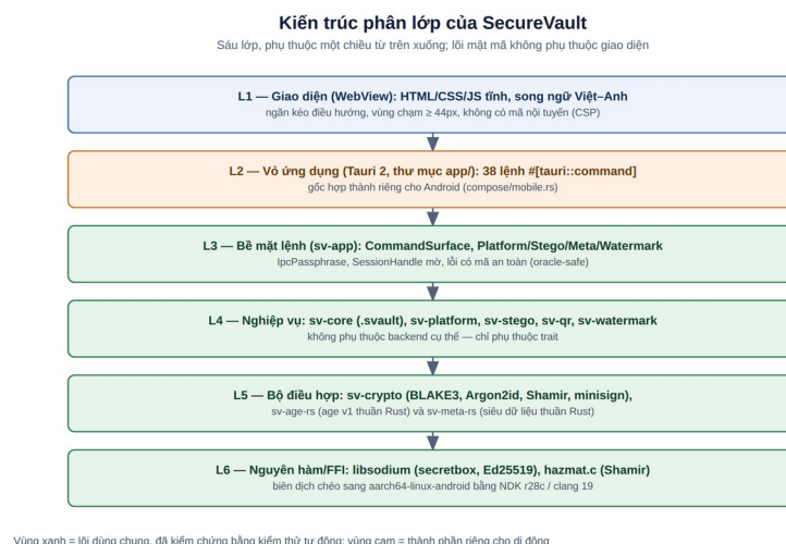
Hình 1. Kiến trúc phân lớp của SecureVault
