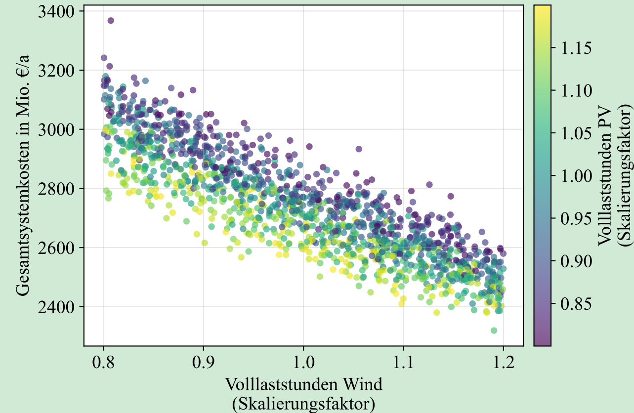
4. Parameterinteraktion Volllaststunden Wind vs. Volllaststunden PV
