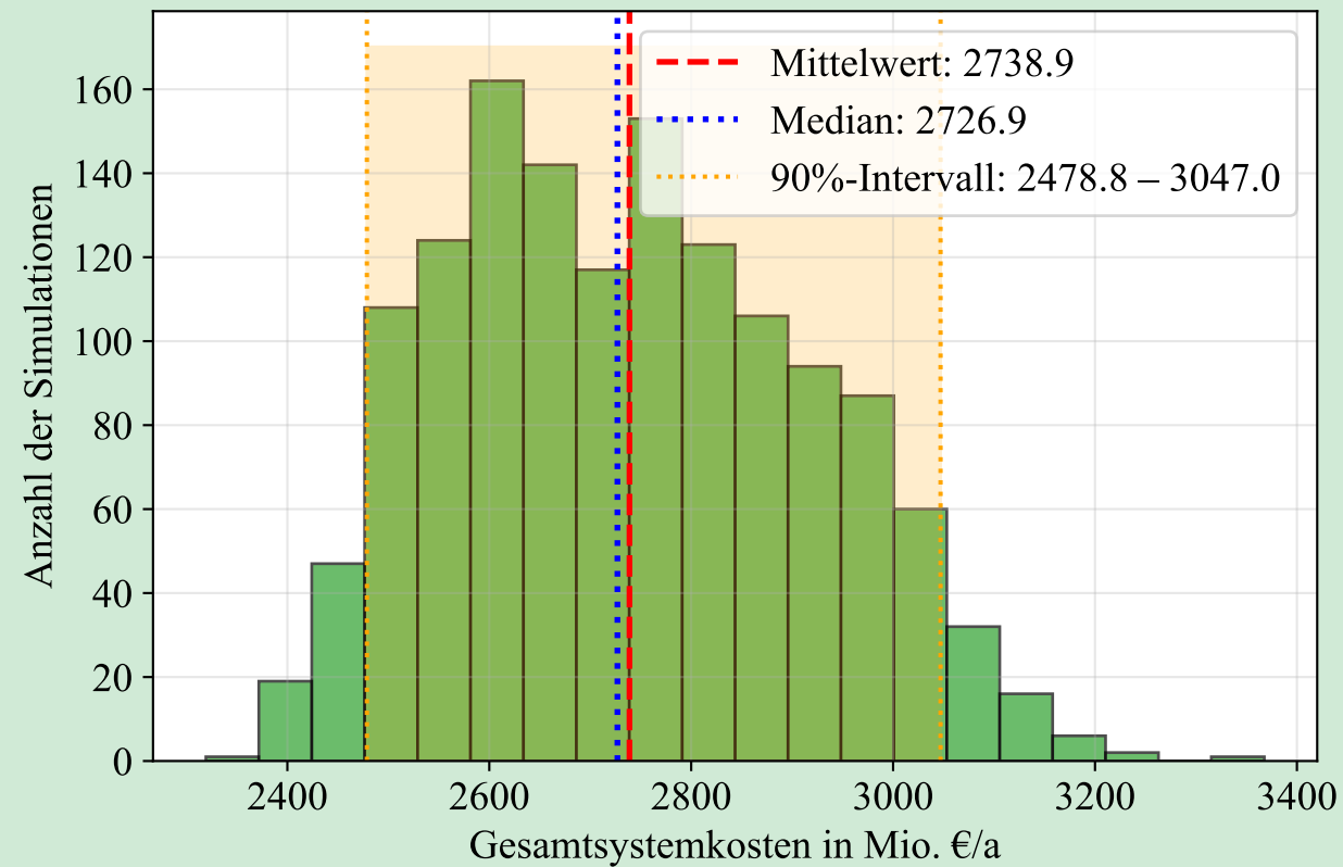
3. Unsicherheit Gesamtsystemkosten aus 1,400 Simulationen
