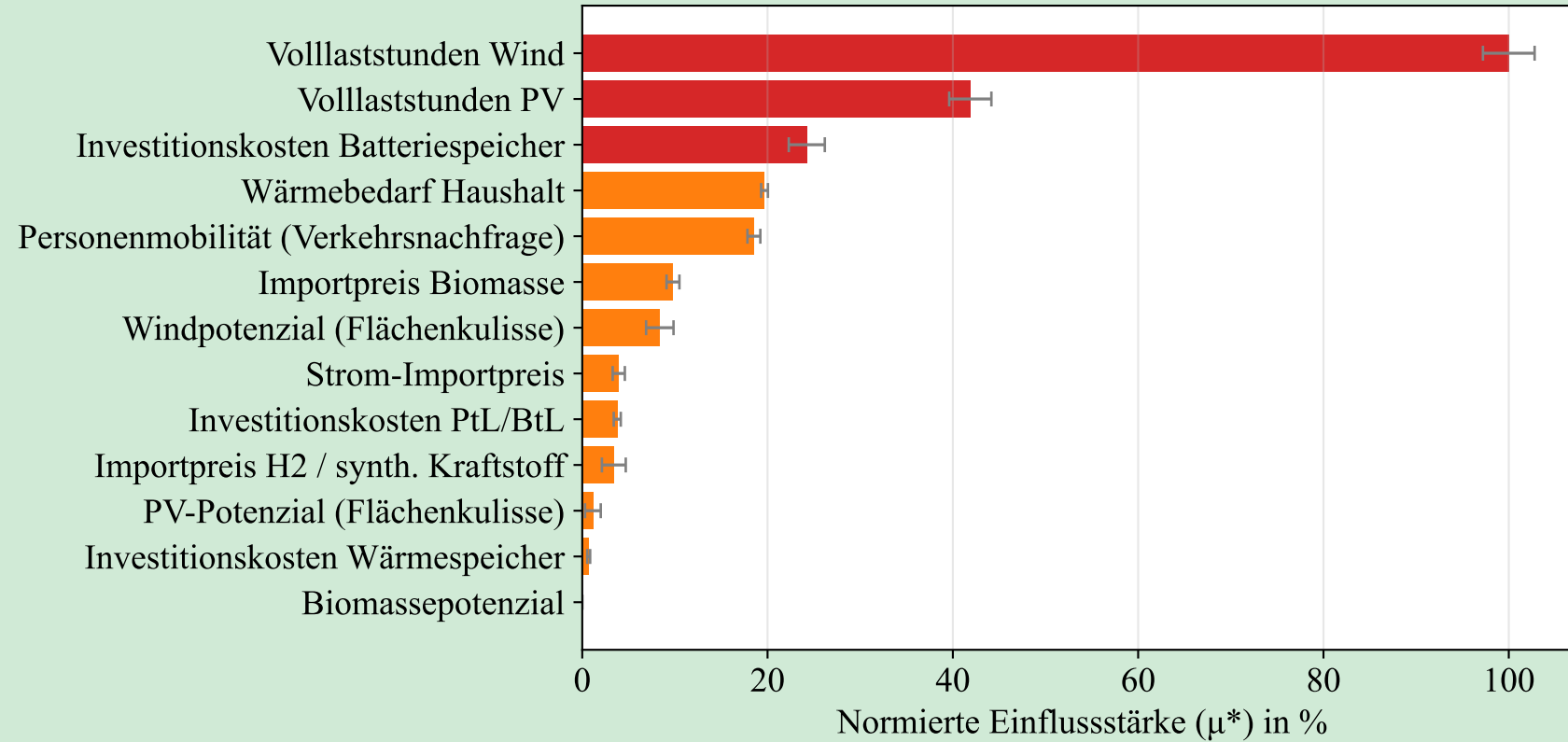
3. Unsicherheit Gesamtsystemkosten aus 1,400 Simulationen
