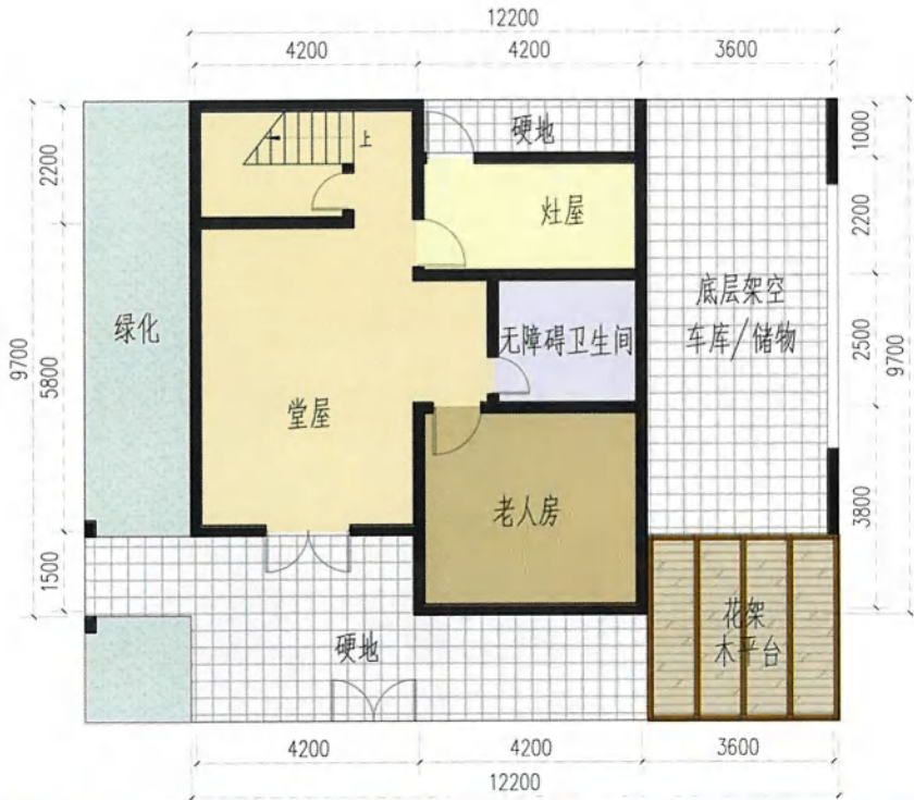
一层平面图
