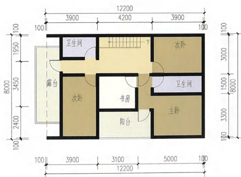
二层平面图
