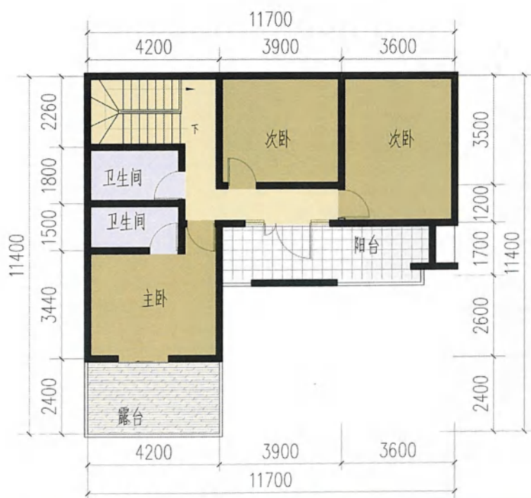
二层平面图
