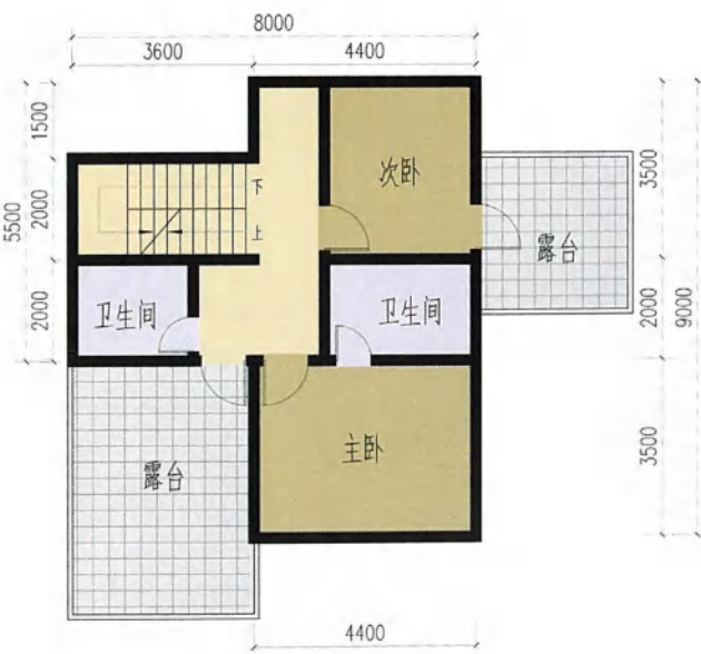
三层平面图
