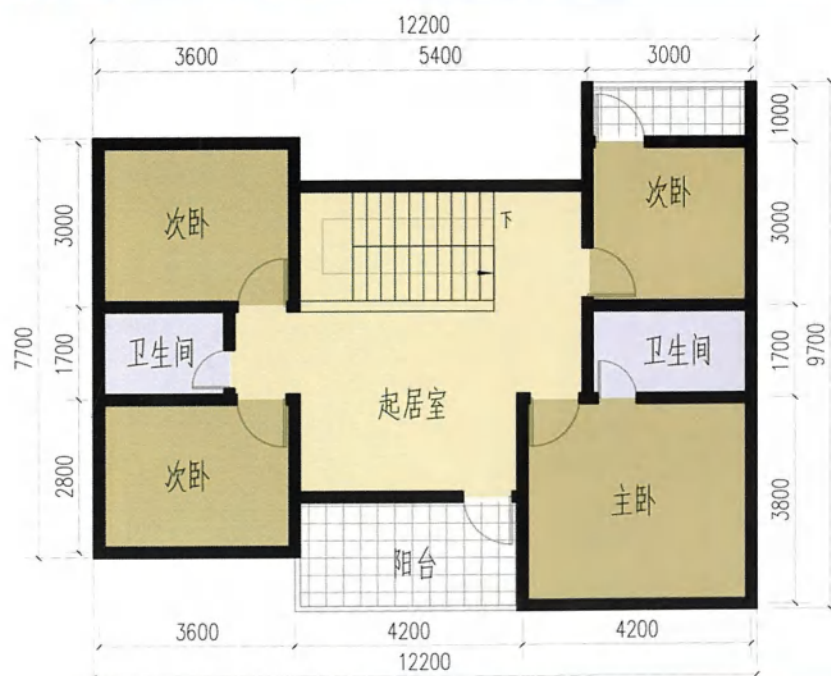
二层平面图
