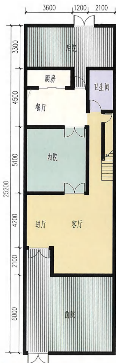
一层平面图
