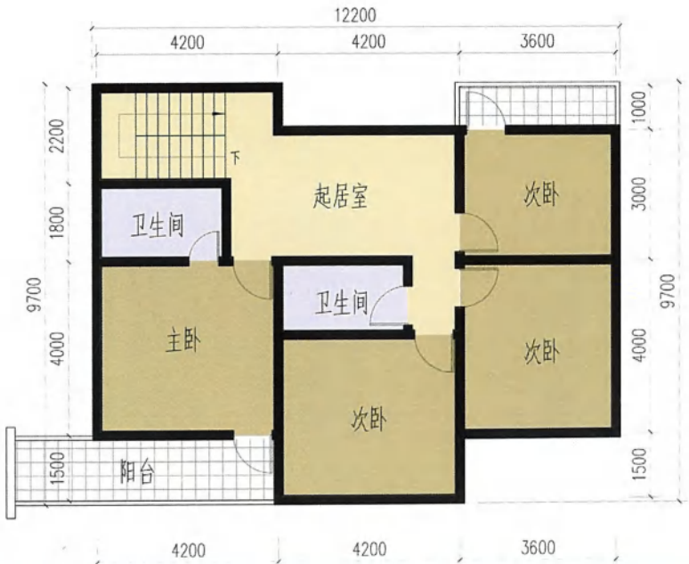
二层平面图
