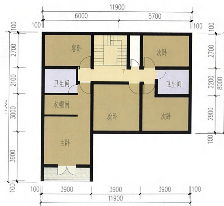
二层平面图
