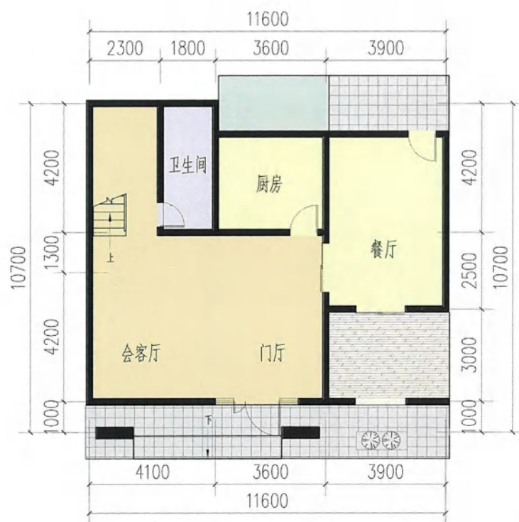
一层平面图
