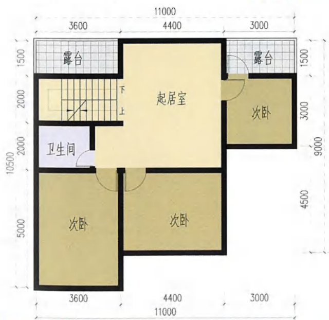
二层平面图
