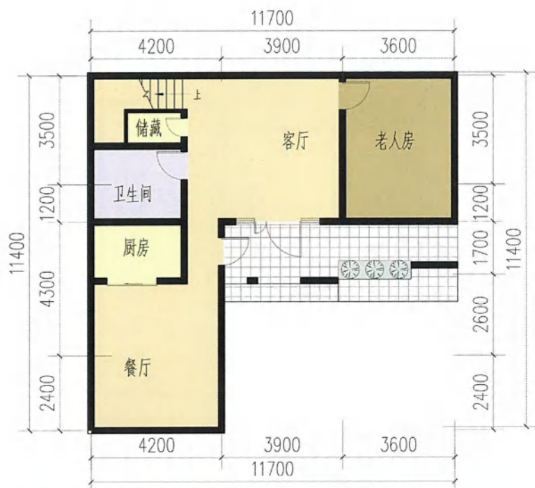
一层平面图
