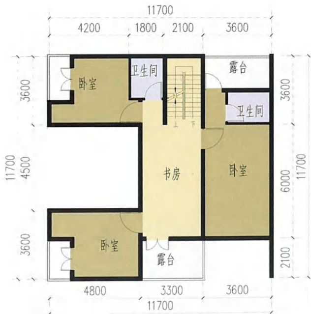
二层平面图 (未加建四人户型)
