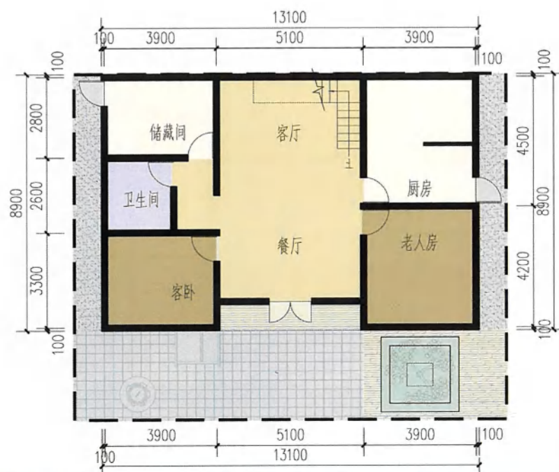
一层平面图
