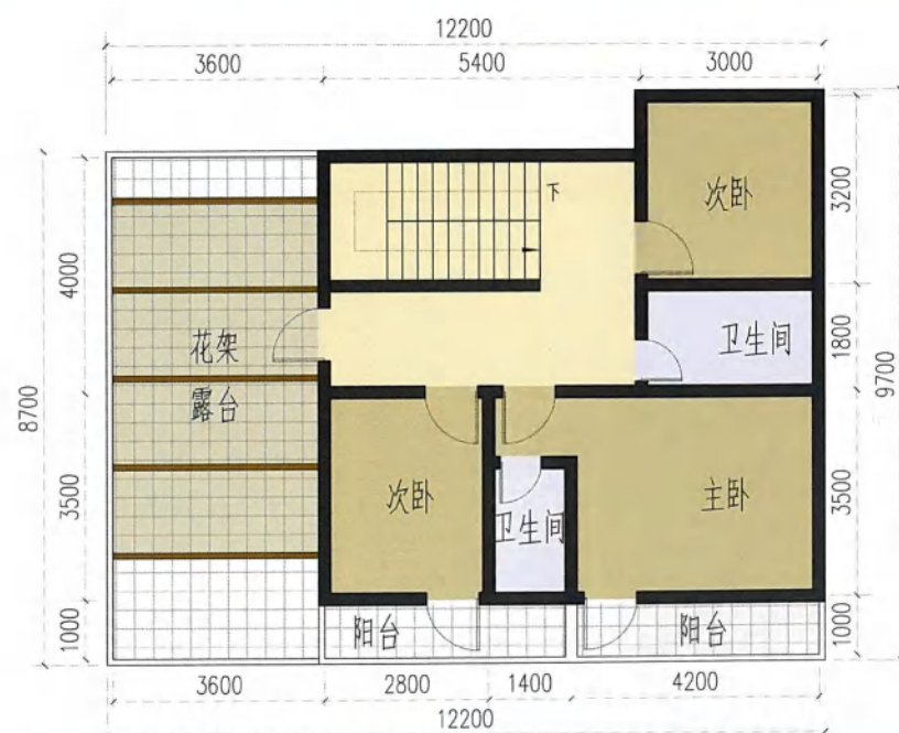
二层平面图
