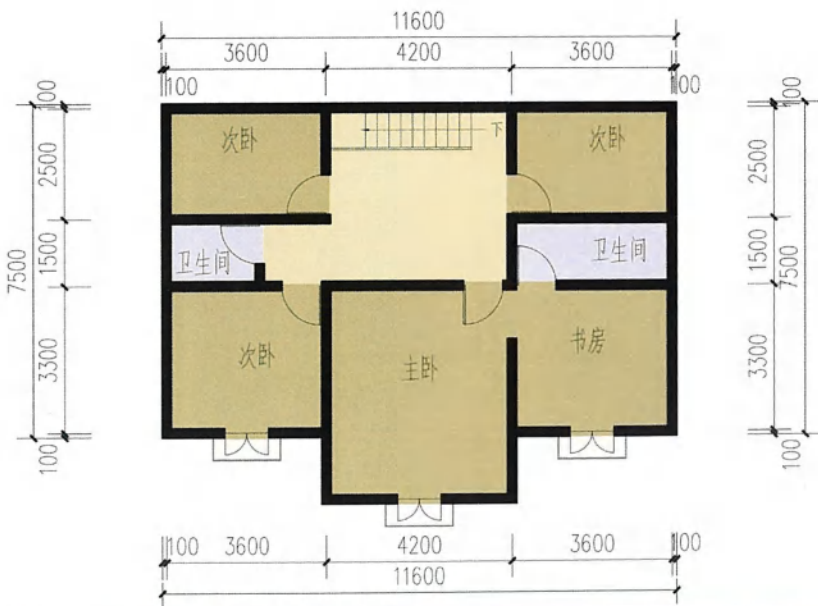
二层平面图
