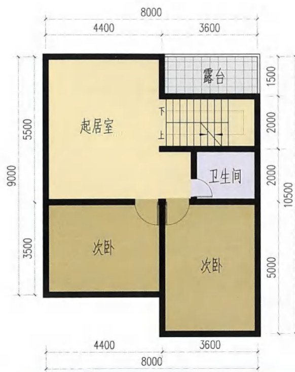
二层平面图
