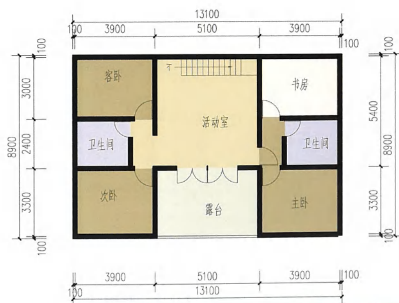
二层平面图
