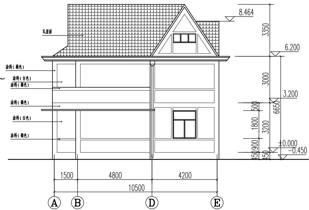
东立面
