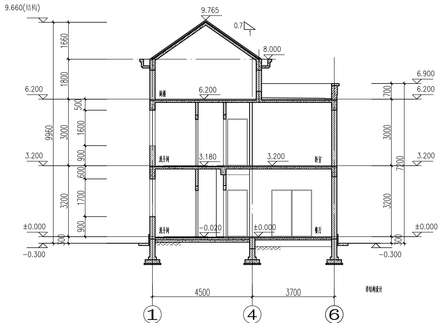
1-1剖面 1:100
