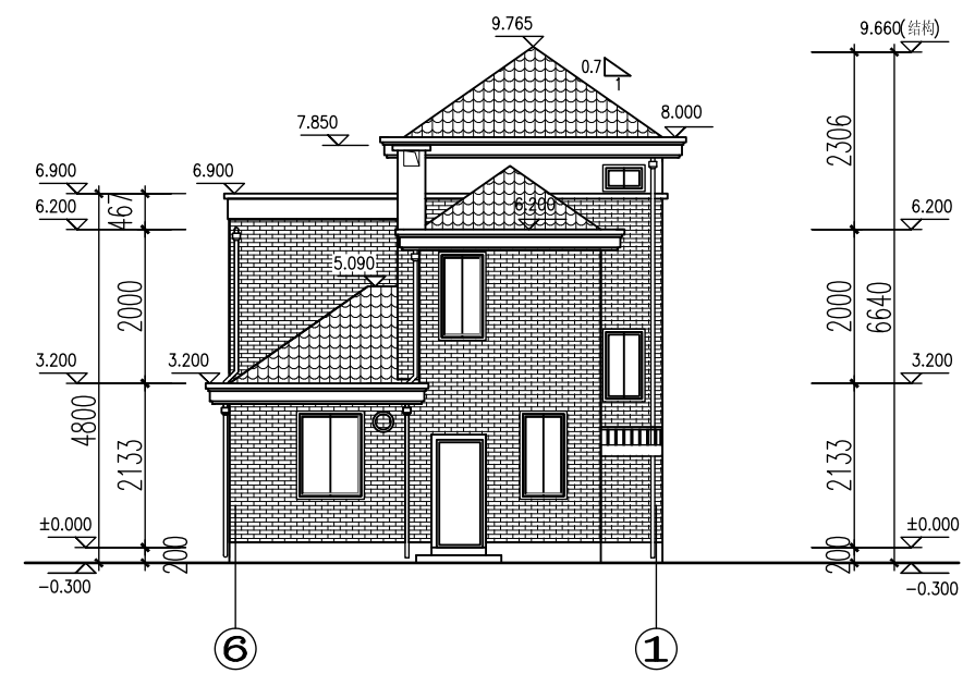
⑥—①轴(北)立面
