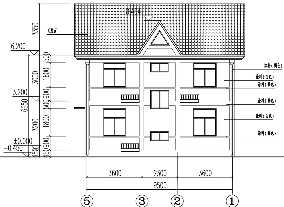
北立面
