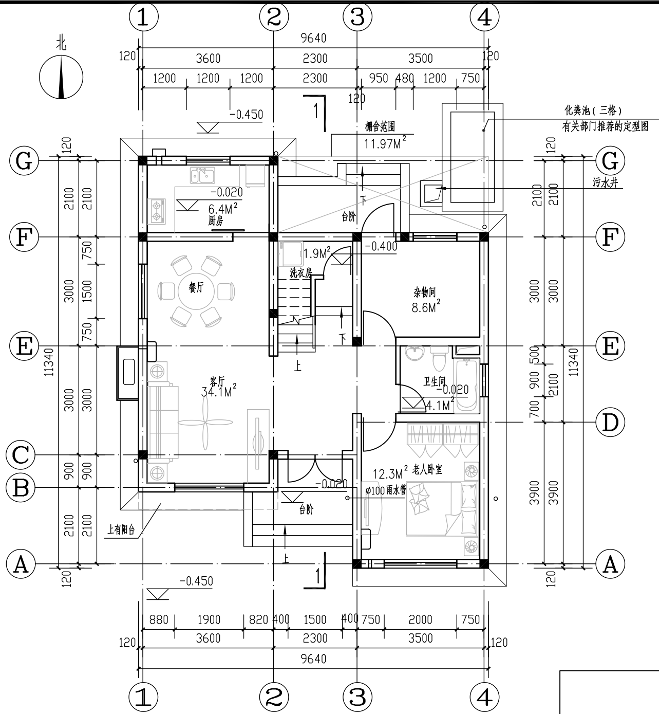
一层平面 1:100
