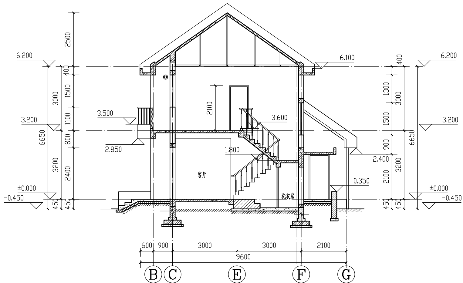
1-1剖面 1:100
