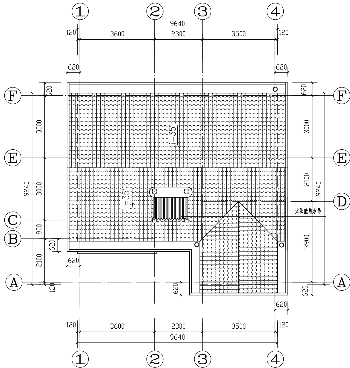
屋顶平面 1:100
