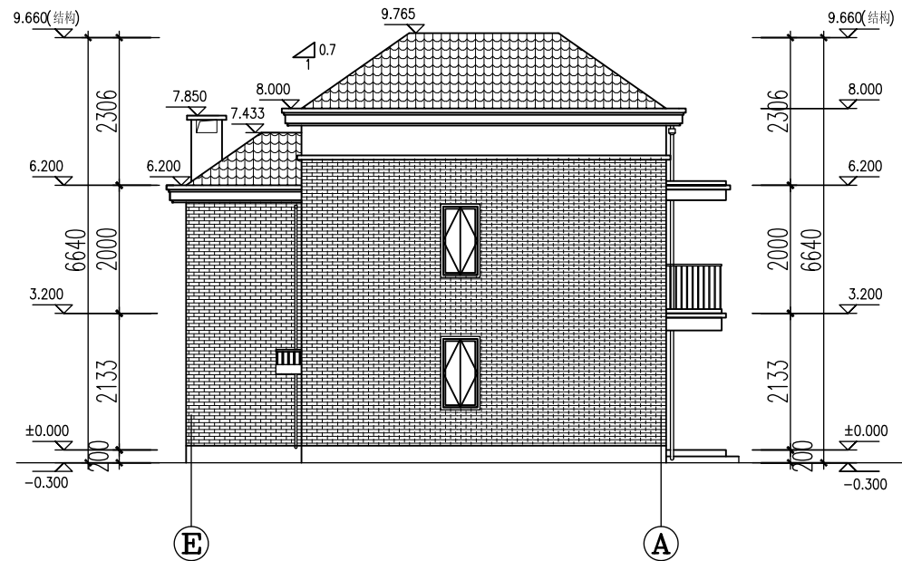
①E—①A轴(西)立面
