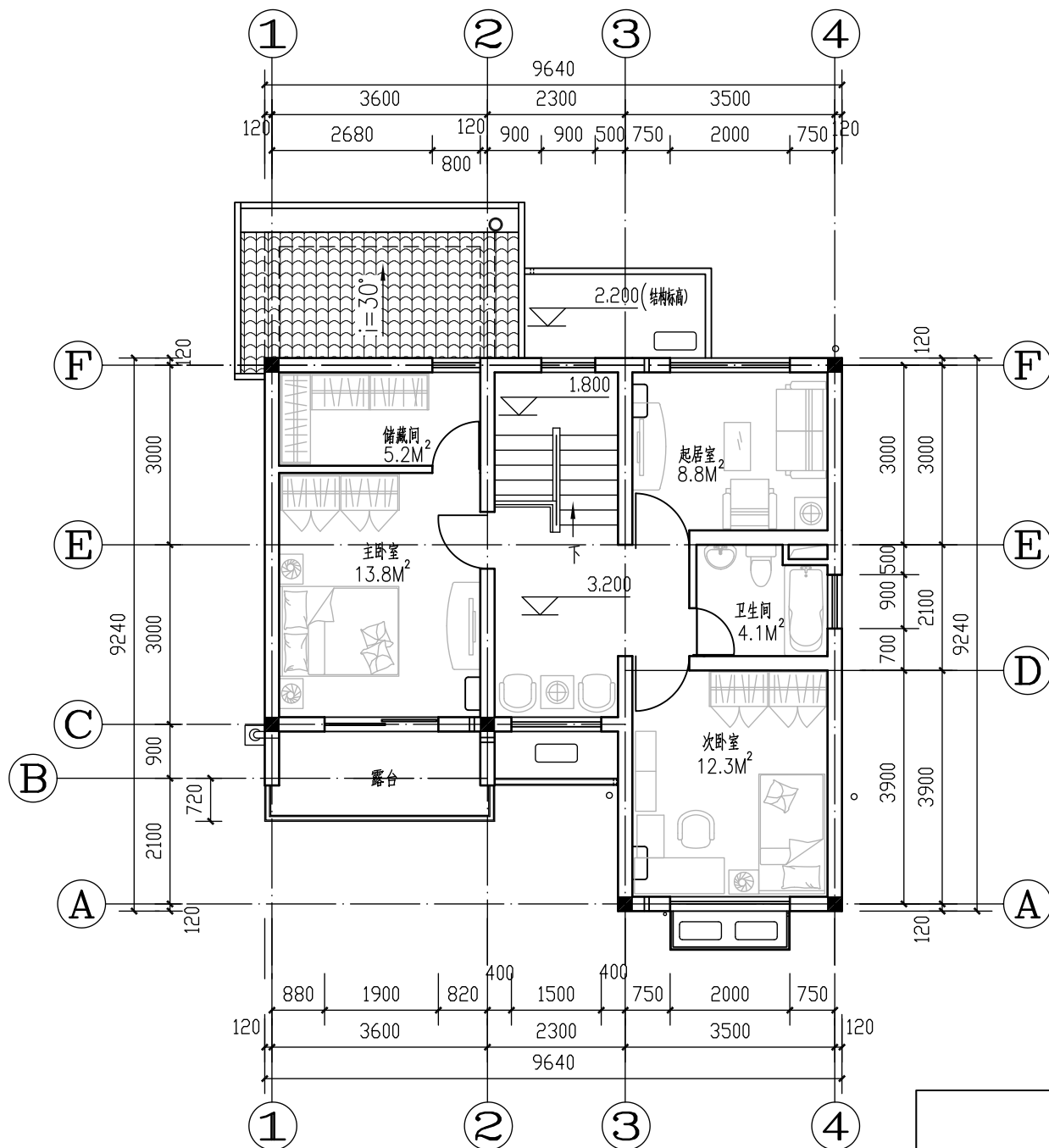
二层平面 1:100
