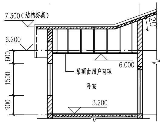
2-2剖面
