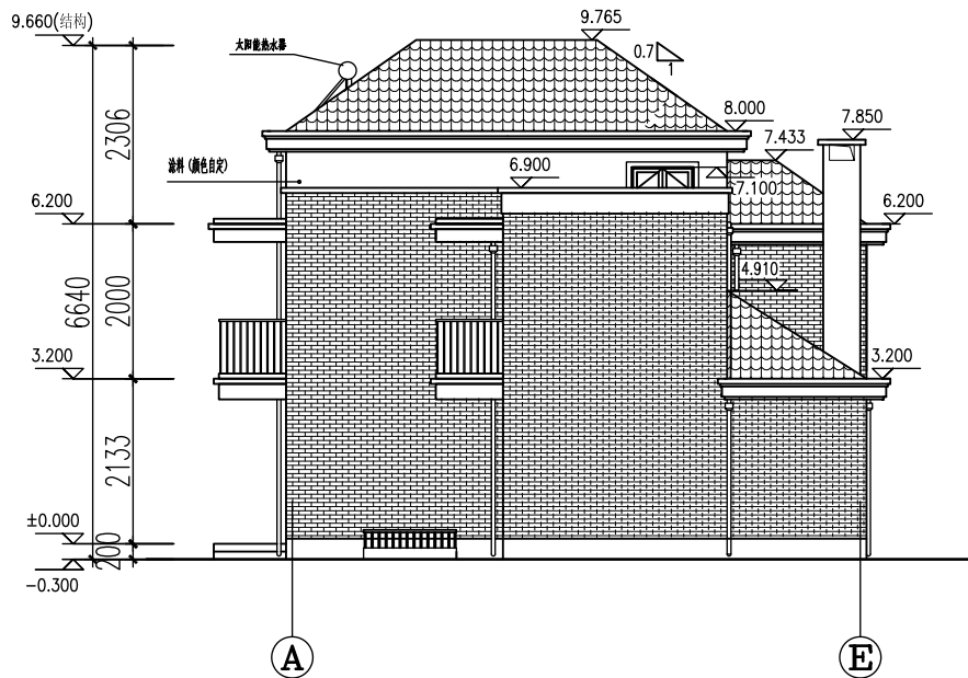
①A—①E轴(东)立面
