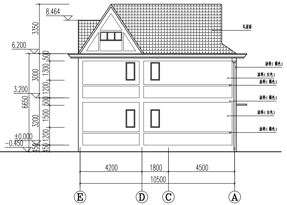
西立面
