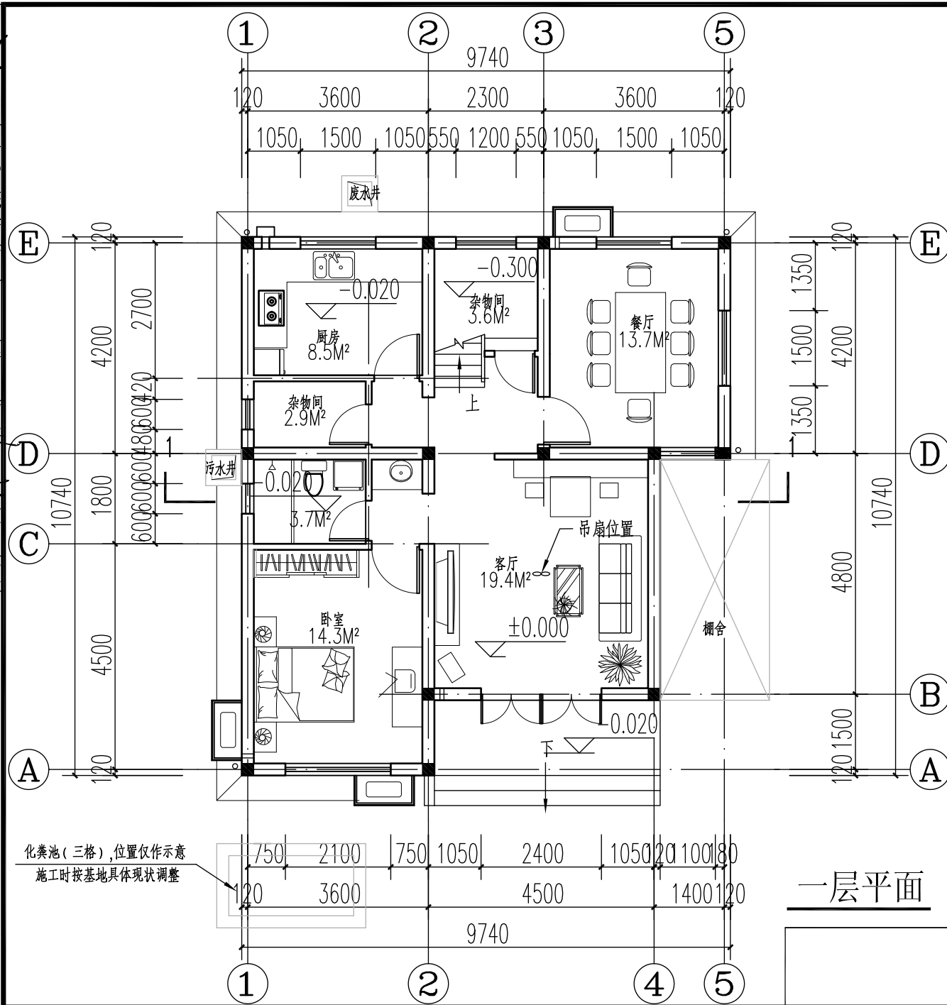
一层平面
