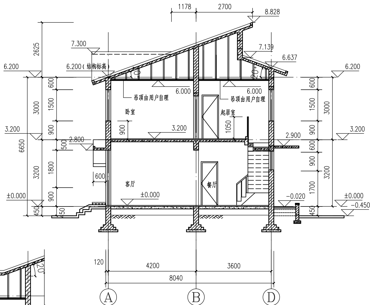
1-1剖面 1:100
