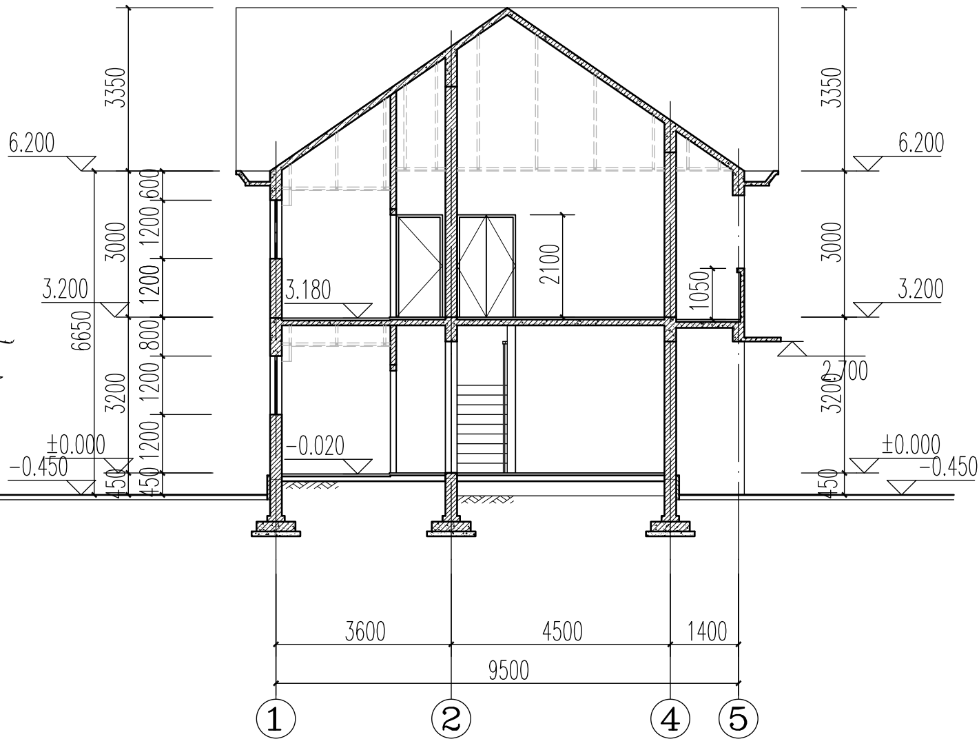
1-1剖面 1:100
