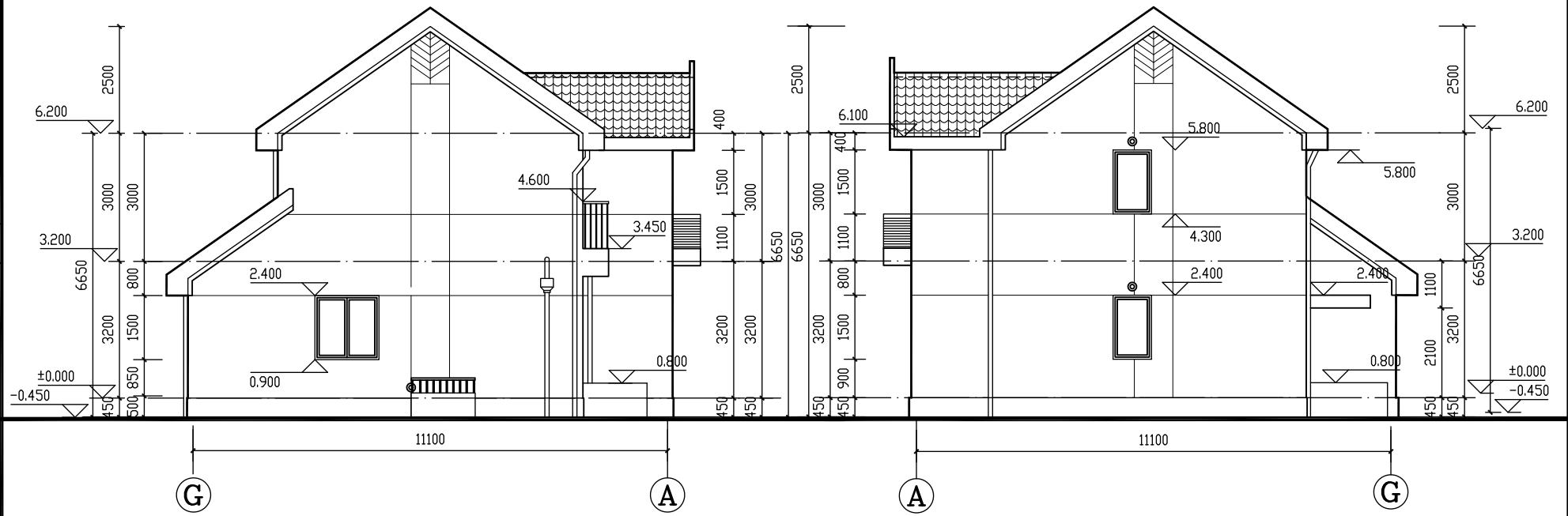
西立面
