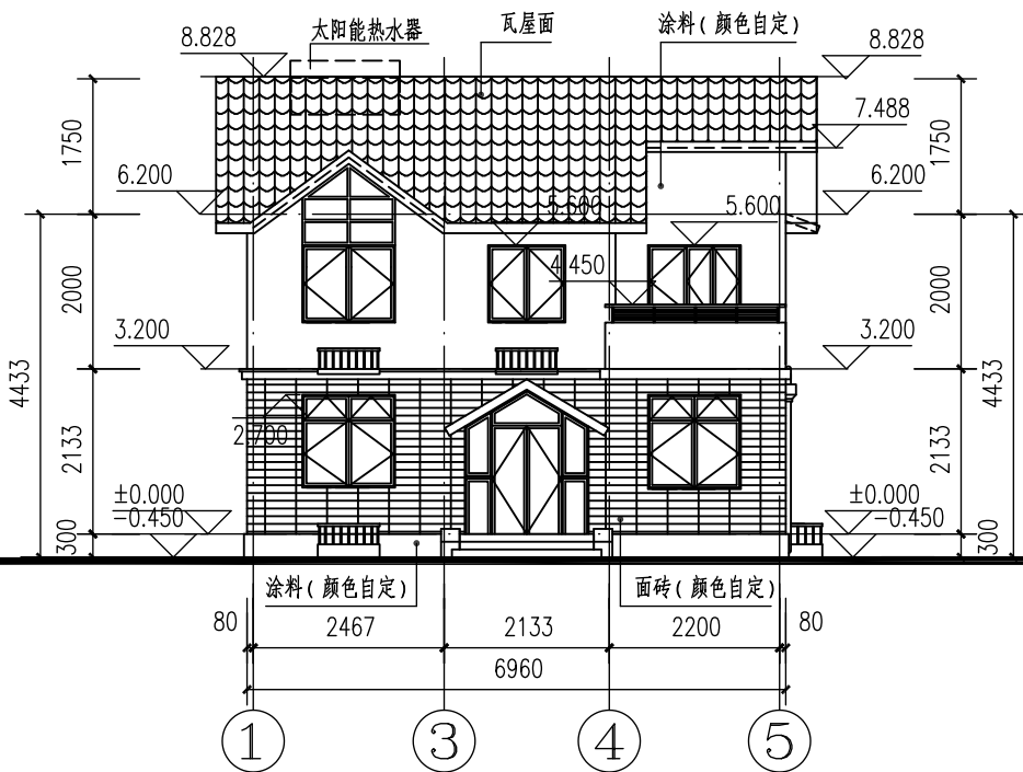
南立面 1:150
