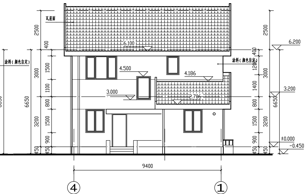
北立面
