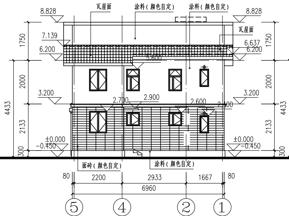
北立面 1:150
