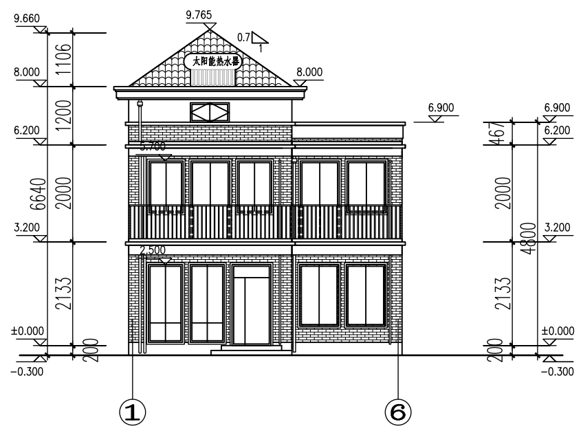
①—⑥轴(南)立面
