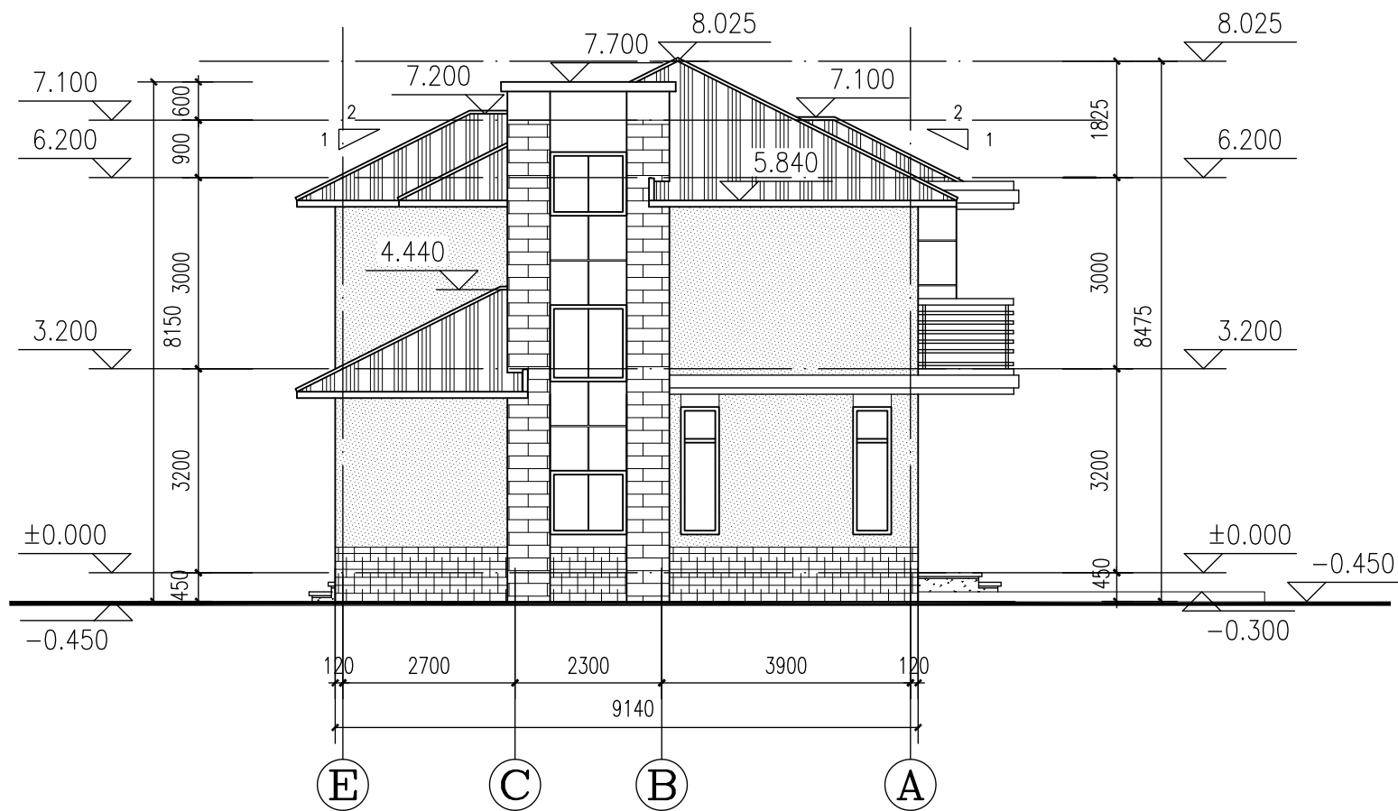
西立面 1:100
