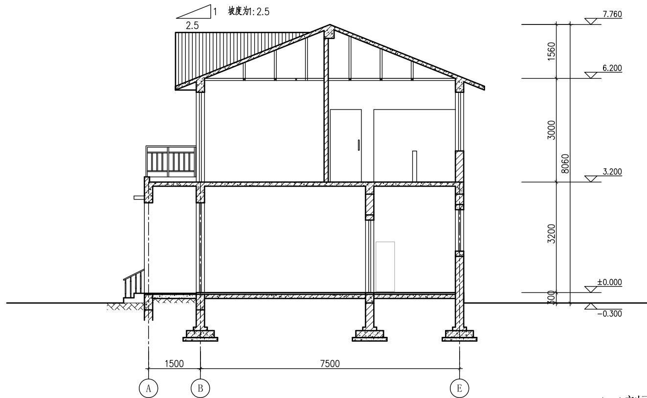
1-1剖面 1:100
