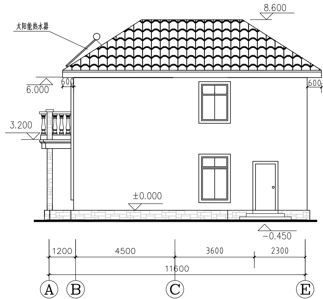
东立面
