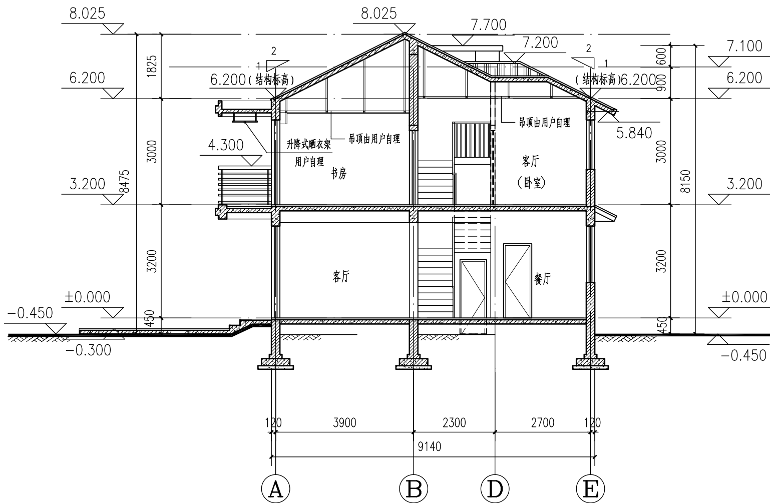
1-1剖面 1:100
