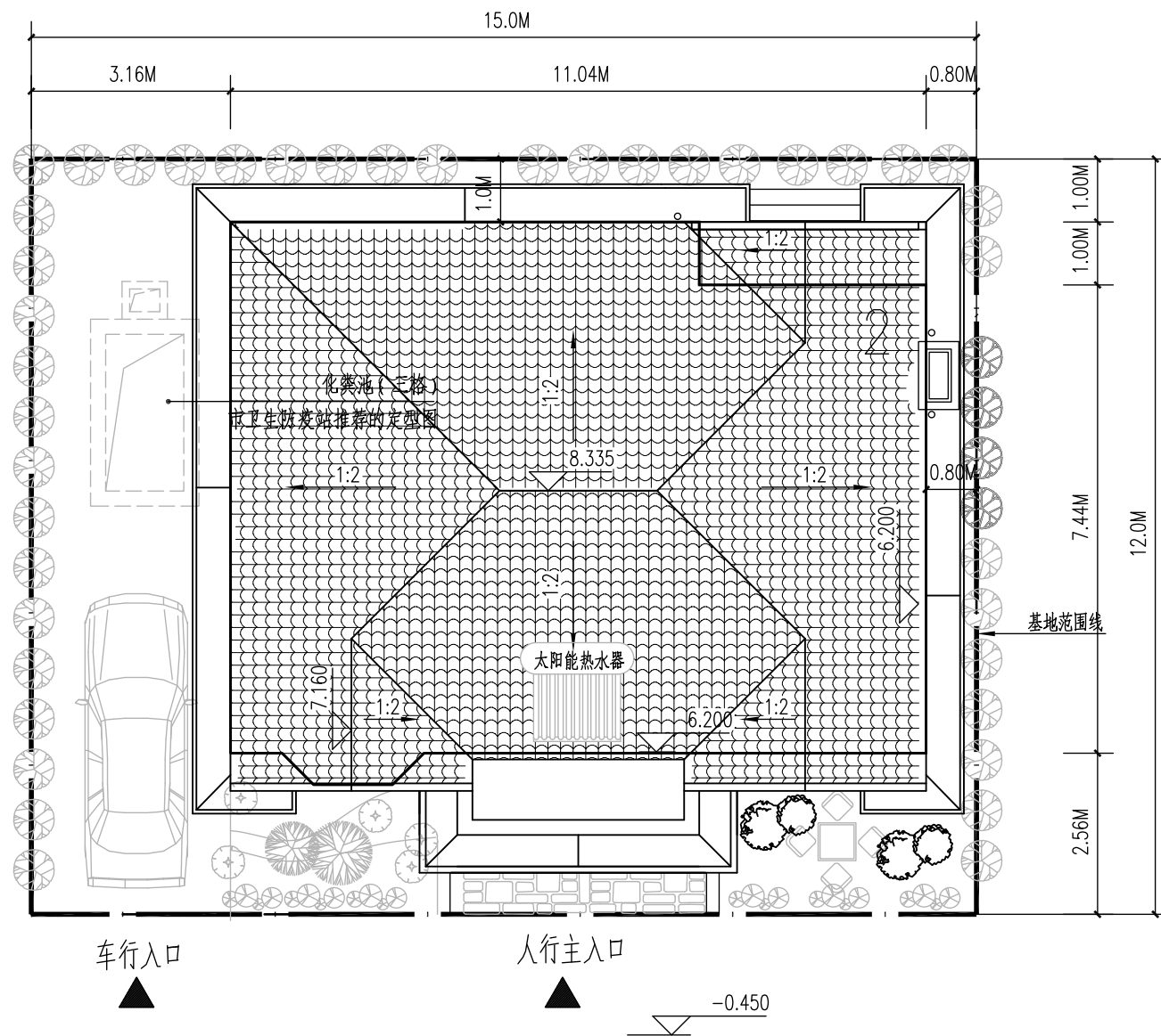
总平面图 1:100
