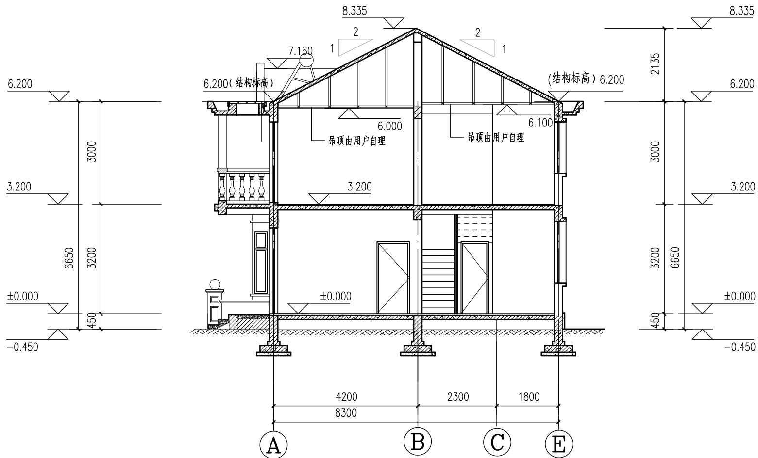
1-1剖面 1:100
