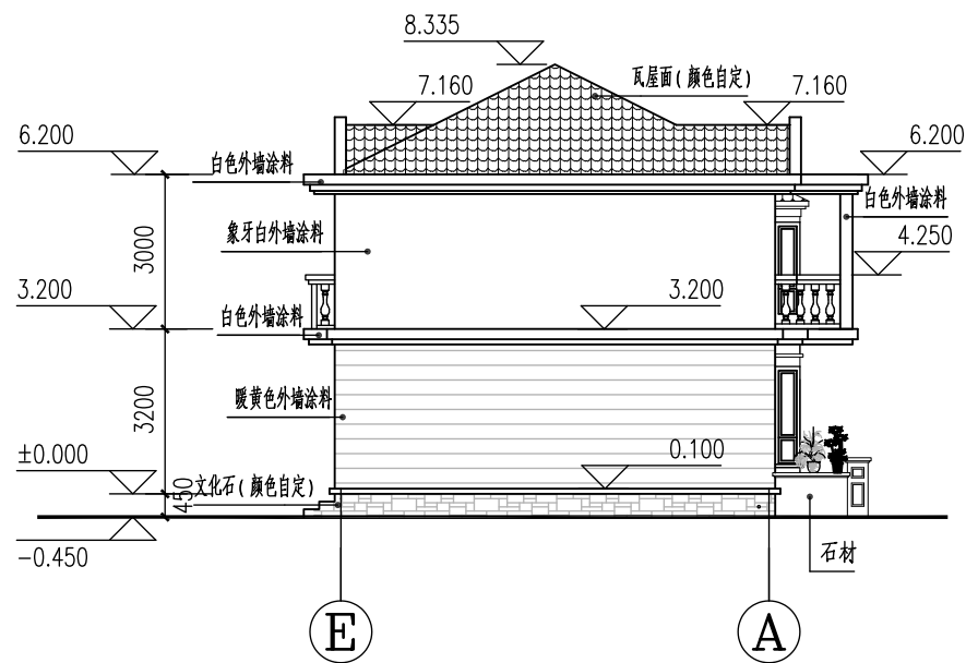
西立面 1:150
