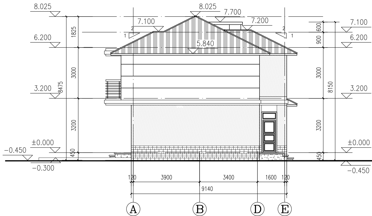
东立面 1:100
