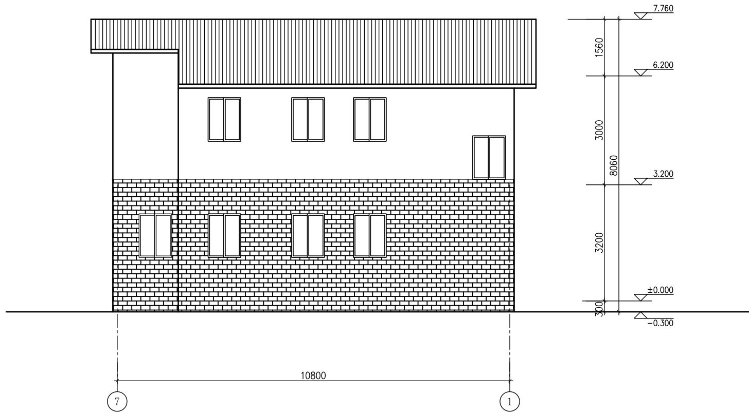
北立面 1:100
