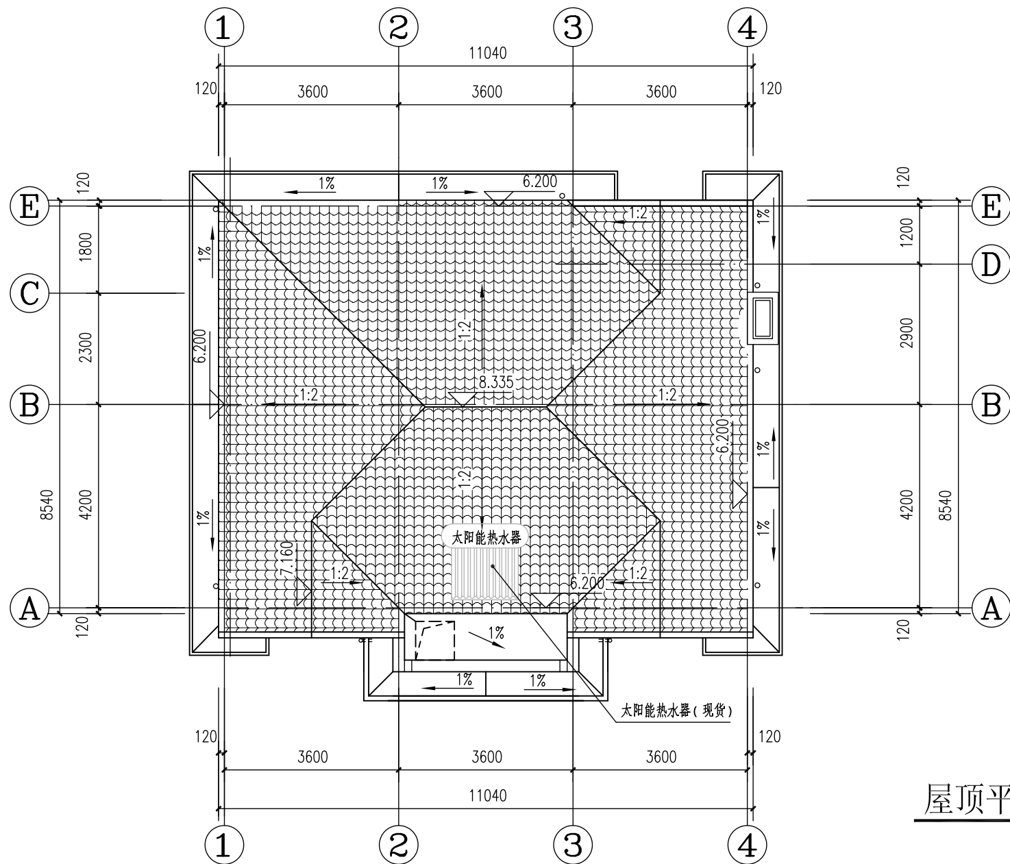
屋顶平面
