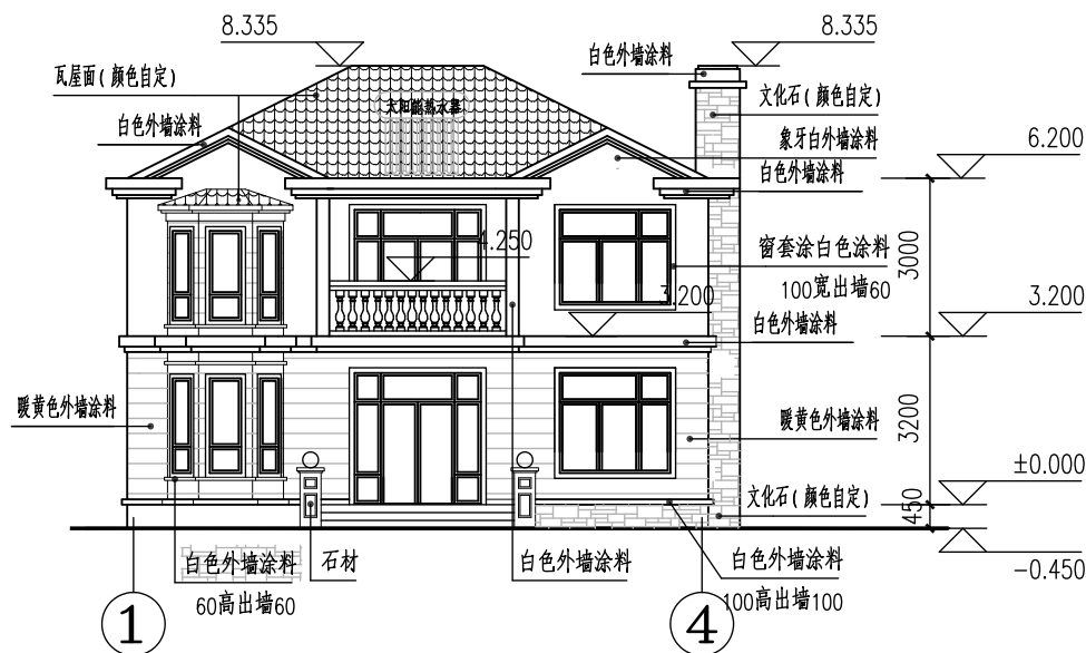
南立面 1:150
