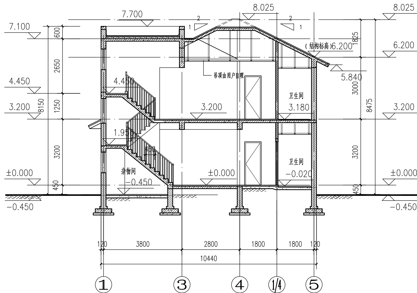
2-2剖面 1:100
