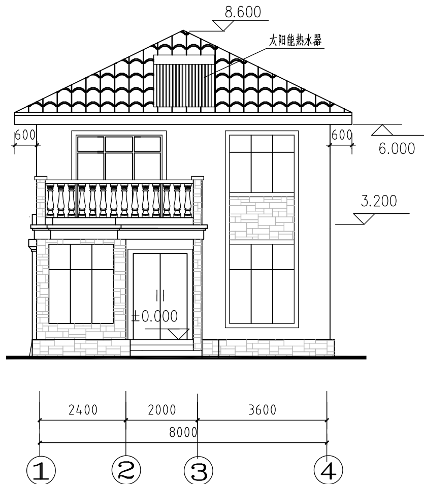
南立面
