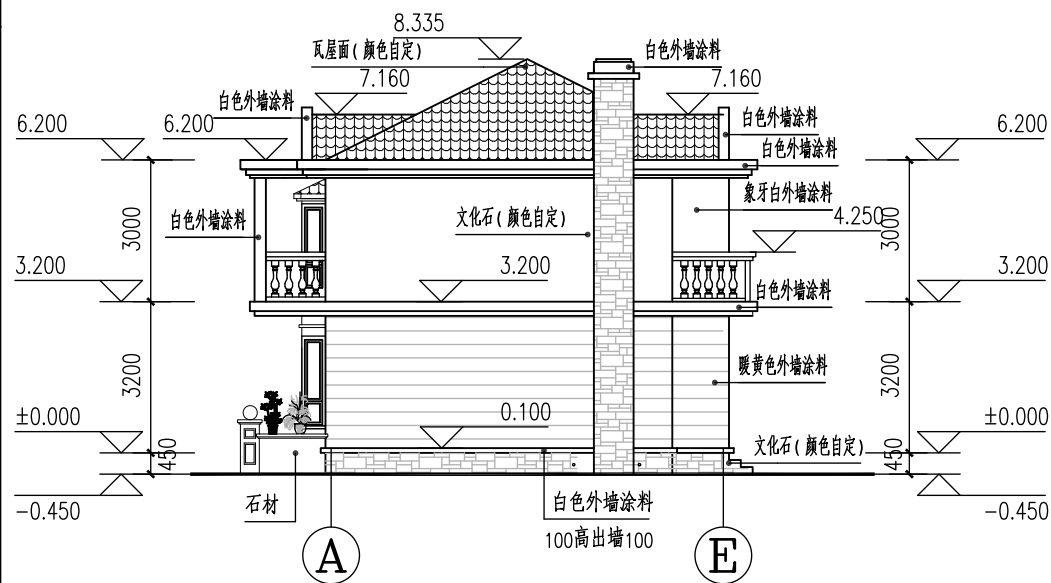
东立面 1:150
